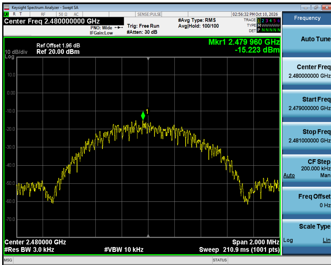
PSD NVNT BLE 1M 2480MHz Ant1
