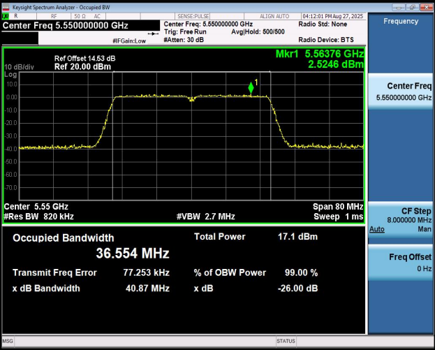
11AC40MIMO-Ant1-5550
