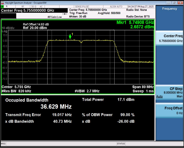
11AC40MIMO-Ant1-5755
