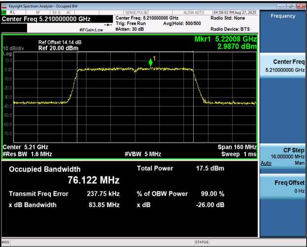
11AC80MIMO-Ant1-5210
