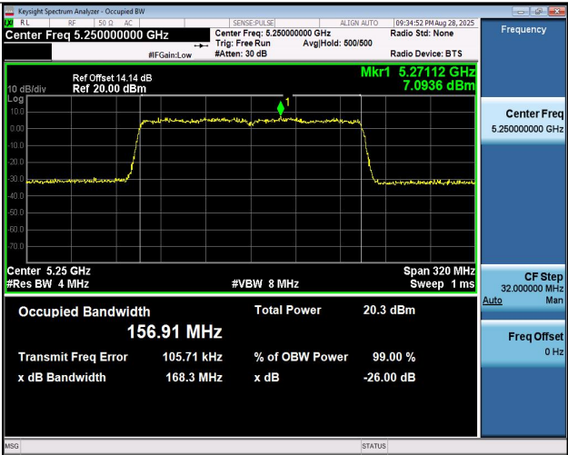
11AX160MIMO-Ant1-5250
