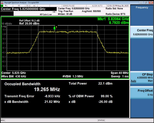
11AX20MIMO-Ant2-5825
