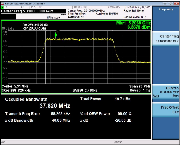
11AX40MIMO-Ant2-5310
