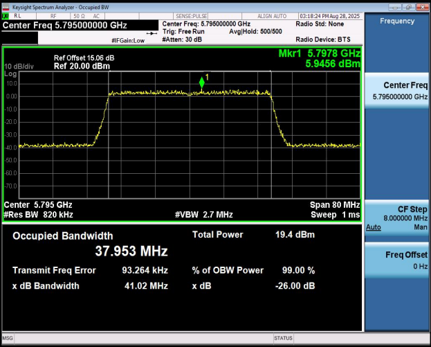
11AX40MIMO-Ant2-5795
