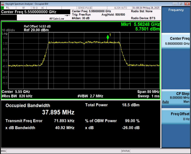
11AX40MIMO-Ant1-5550
