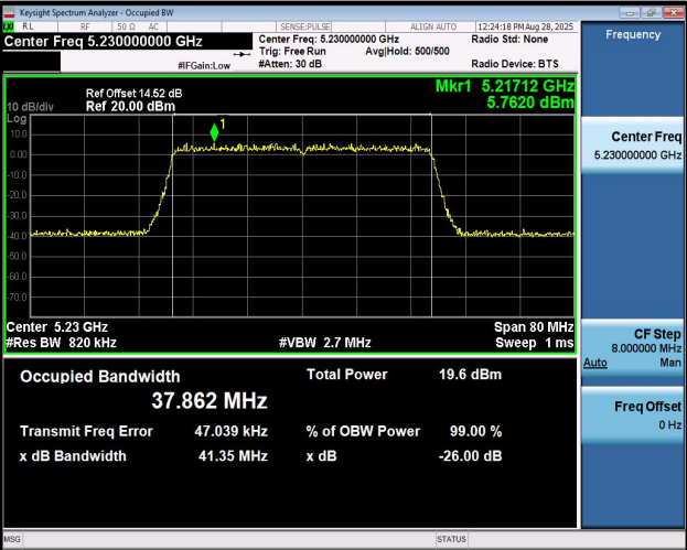
11AX40MIMO-Ant2-5230
