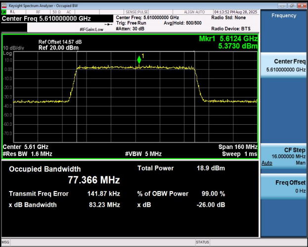
11AX80MIMO-Ant1-5610
