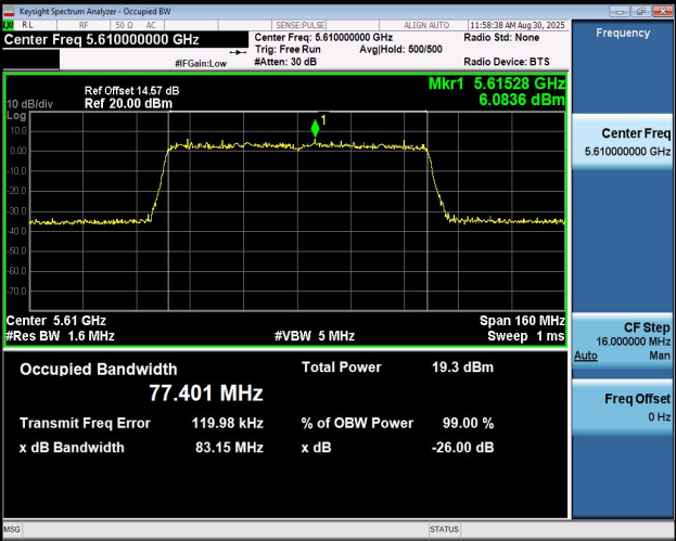
11BE80MIMO-Ant1-5610
