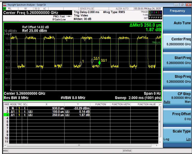
NTNV-11N20MIMO-Ant2-5260
