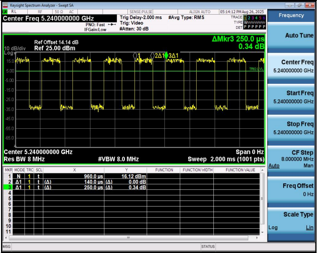
NTNV-11N20MIMO-Ant1-5240
