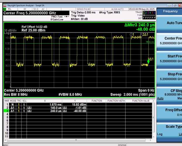
NTNV-11N20MIMO-Ant1-5200
