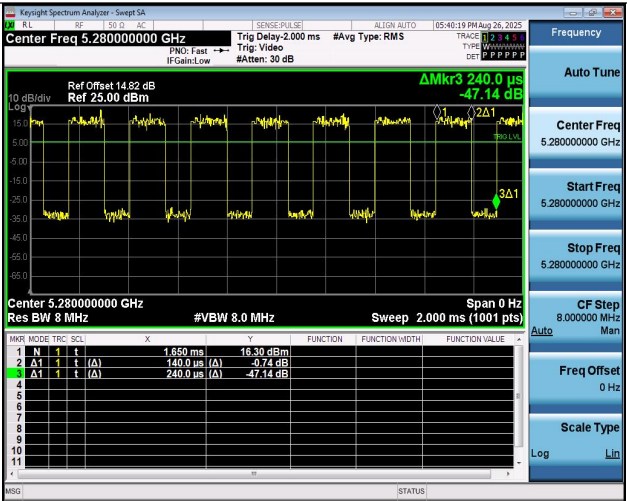
NTNV-11N20MIMO-Ant2-5280
