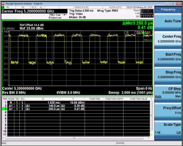
NTNV-11N20MIMO-Ant2-5200
