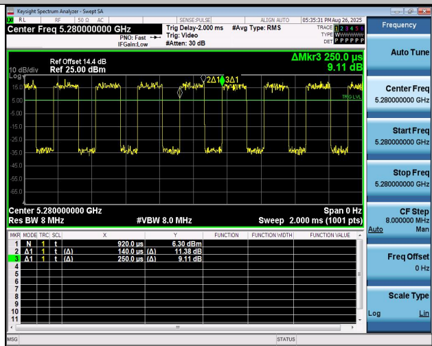
NTNV-11N20MIMO-Ant1-5280
