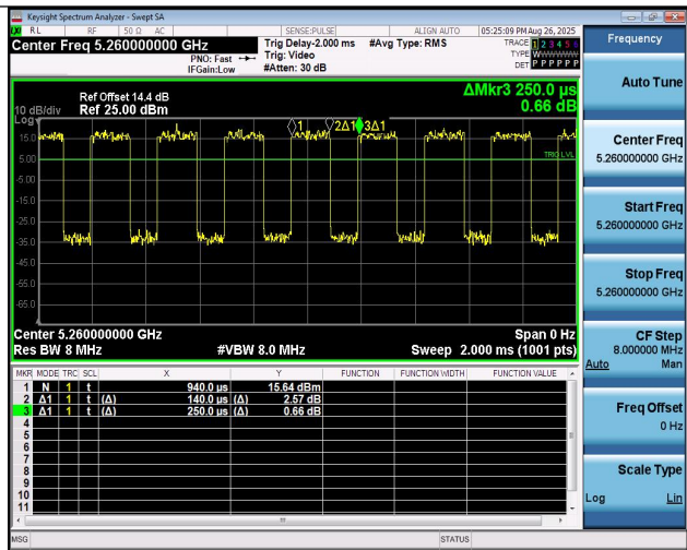
NTNV-11N20MIMO-Ant1-5260
