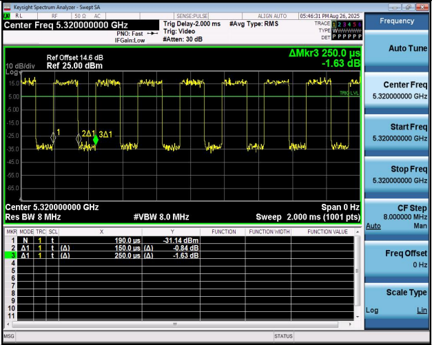
NTNV-11N20MIMO-Ant1-5320
