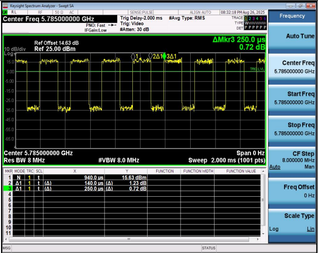
NTNV-11N20MIMO-Ant1-5785
