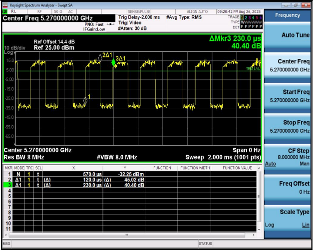
NTNV-11N40MIMO-Ant1-5270
