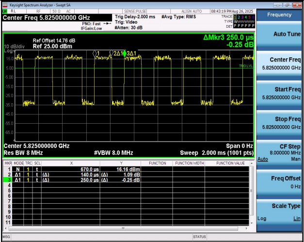
NTNV-11N20MIMO-Ant1-5825
