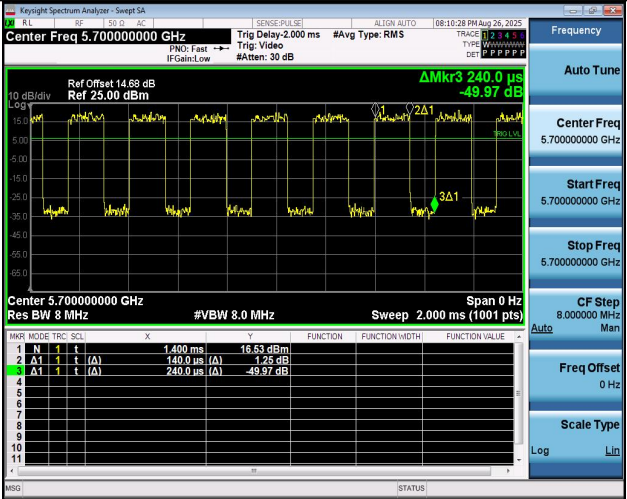
NTNV-11N20MIMO-Ant1-5700
