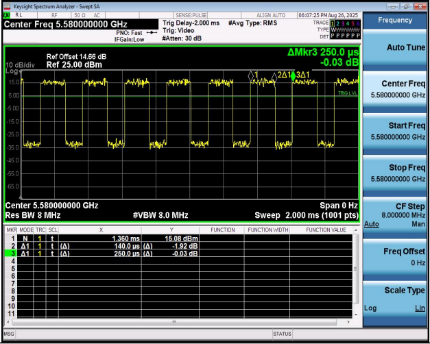
NTNV-11N20MIMO-Ant1-5580
