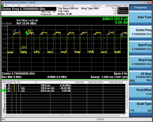
NTNV-11N40MIMO-Ant1-5795
