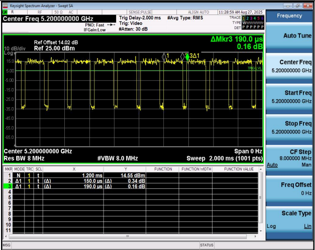
NTNV-11AC20MIMO-Ant1-5200
