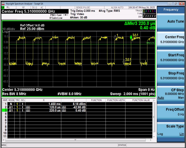
NTNV-11N40MIMO-Ant1-5310
