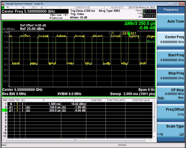
NTNV-11N20MIMO-Ant1-5500
