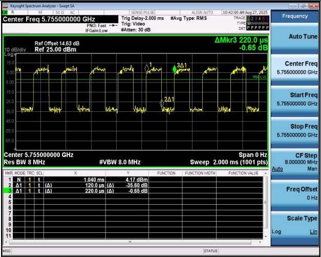
NTNV-11N40MIMO-Ant1-5755
