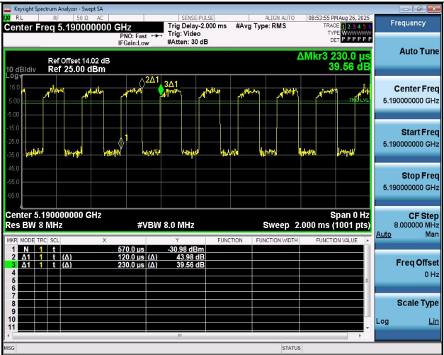
NTNV-11N40MIMO-Ant1-5190
