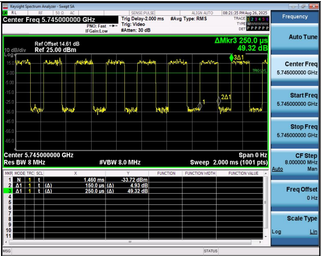
NTNV-11N20MIMO-Ant1-5745
