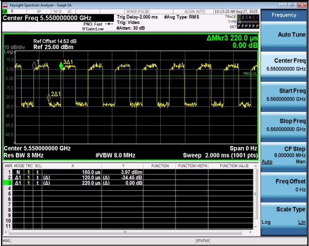
NTNV-11N40MIMO-Ant1-5550
