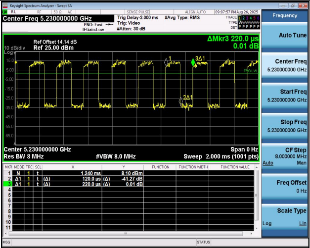
NTNV-11N40MIMO-Ant1-5230
