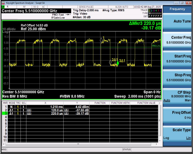
NTNV-11N40MIMO-Ant1-5510
