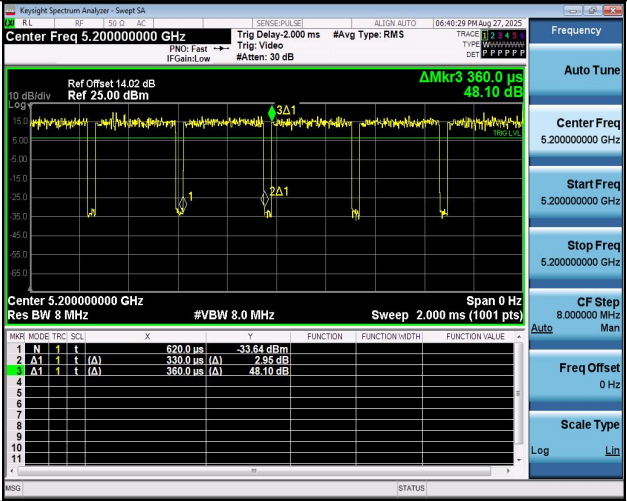
NTNV-11AX20MIMO-Ant1-5200
