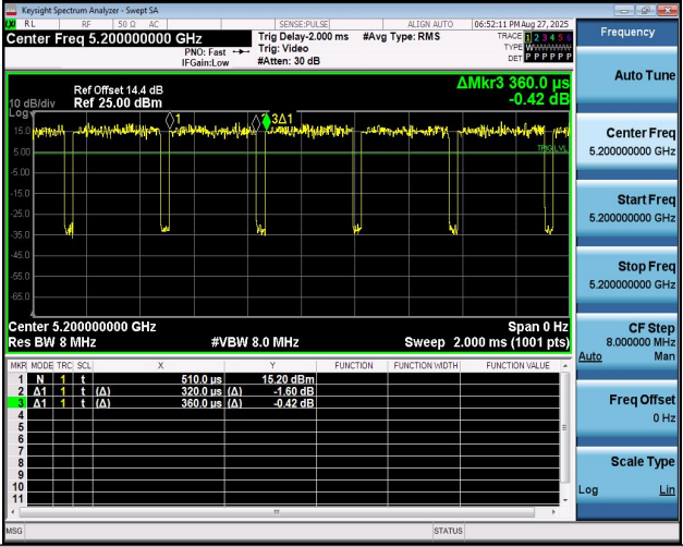
NTNV-11AX20MIMO-Ant2-5200
