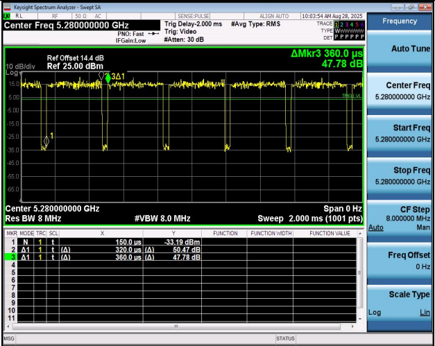
NTNV-11AX20MIMO-Ant1-5280
