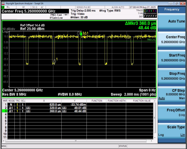
NTNV-11AX20MIMO-Ant1-5260
