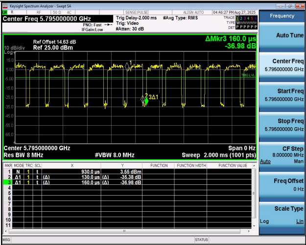
NTNV-11AC40MIMO-Ant1-5795
