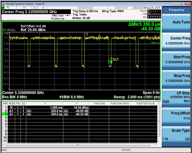
NTNV-11AX20MIMO-Ant1-5320
