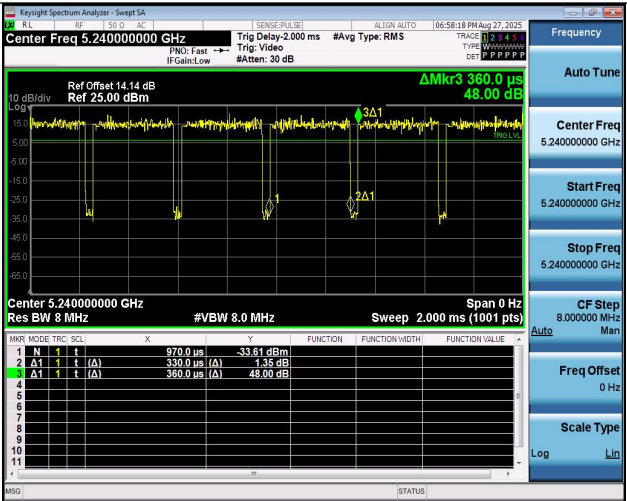
NTNV-11AX20MIMO-Ant1-5240
