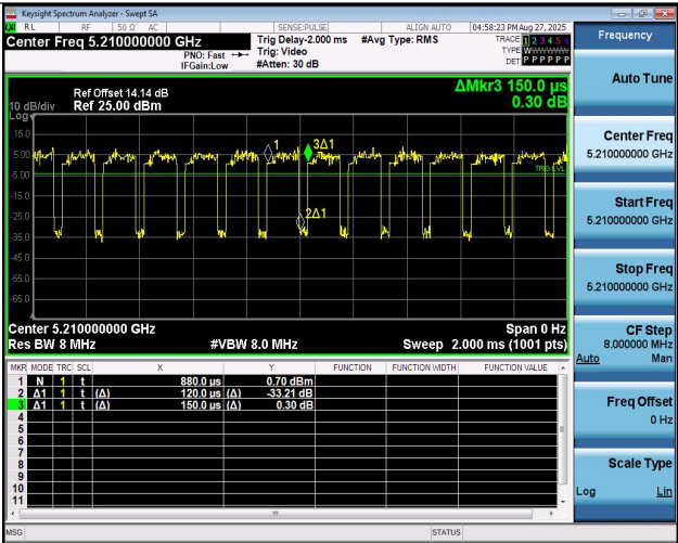
NTNV-11AC80MIMO-Ant1-5210
