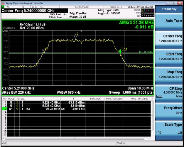
11N20MIMO-Ant1-5240
