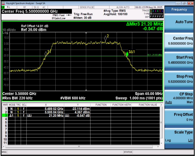
11N20MIMO-Ant2-5500
