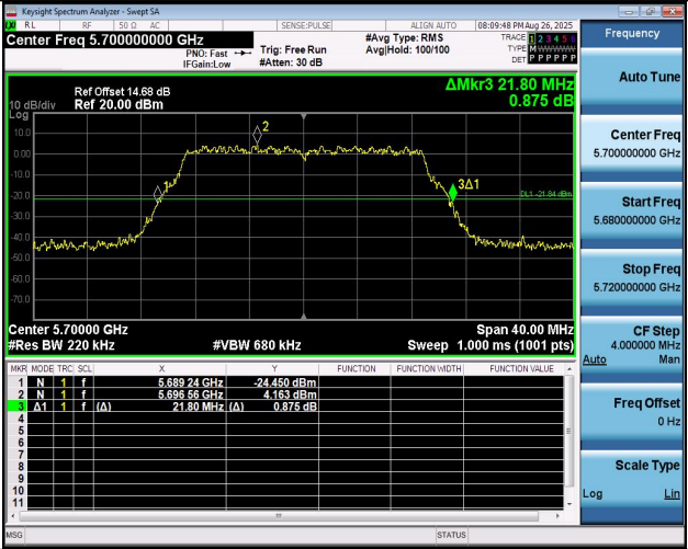
11N20MIMO-Ant1-5700
