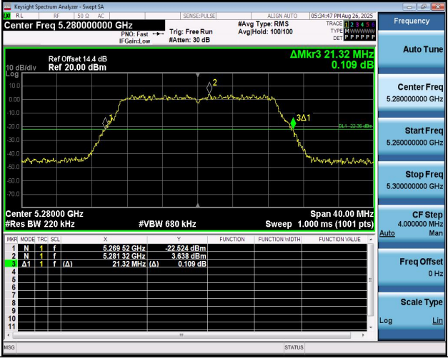
11N20MIMO-Ant1-5280
