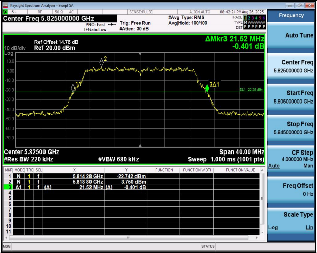
11N20MIMO-Ant1-5825
