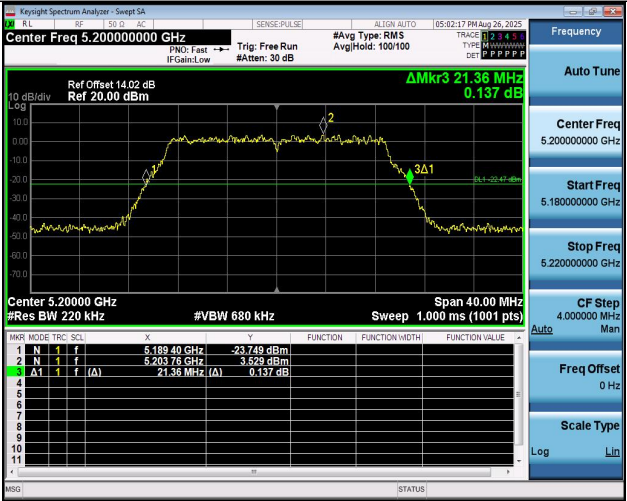
11N20MIMO-Ant1-5200
