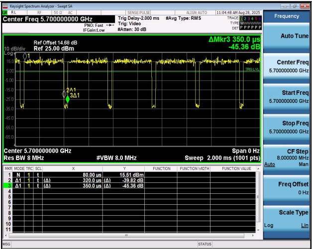
NTNV-11AX20MIMO-Ant1-5700
