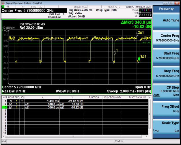
NTNV-11AX40MIMO-Ant2-5795
