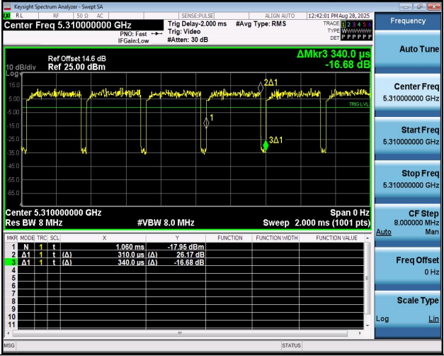
NTNV-11AX40MIMO-Ant1-5310
