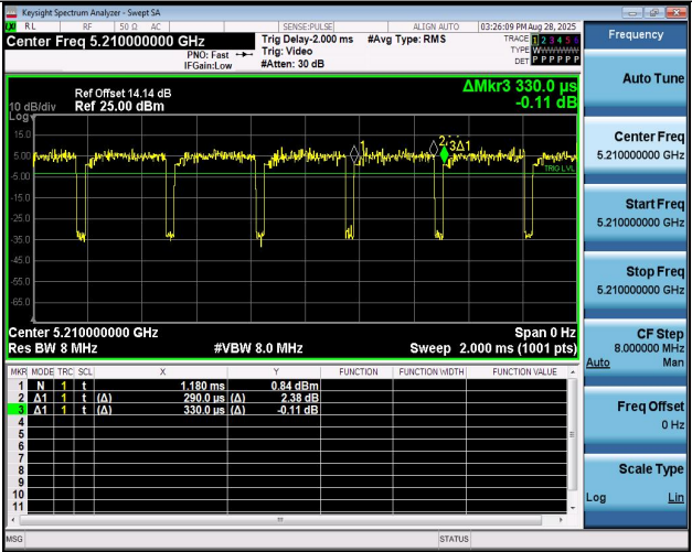
NTNV-11AX80MIMO-Ant1-5210
