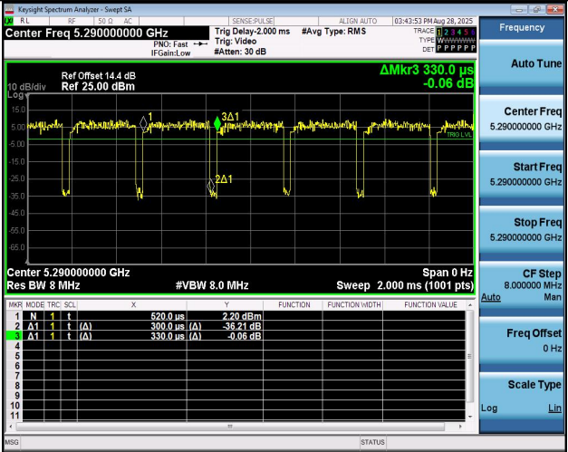
NTNV-11AX80MIMO-Ant1-5290
