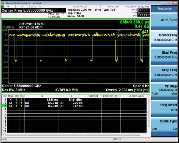
NTNV-11AX20MIMO-Ant1-5580
