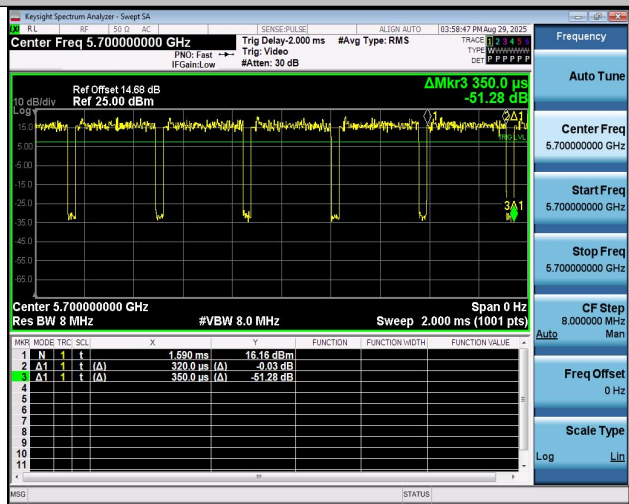
NTNV-11BE20MIMO-Ant1-5700
