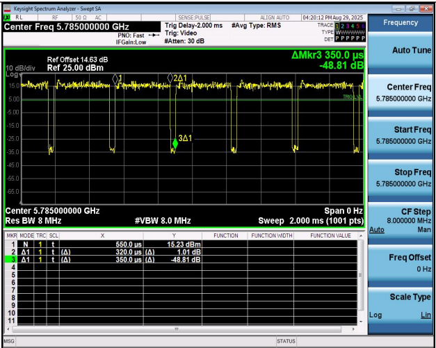
NTNV-11BE20MIMO-Ant1-5785
