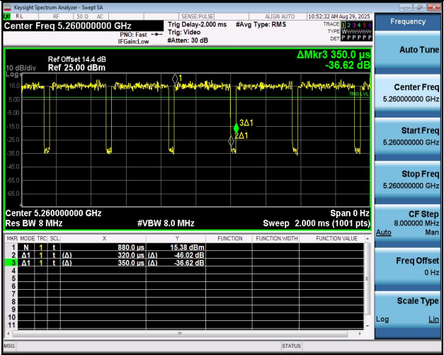
NTNV-11BE20MIMO-Ant1-5260
