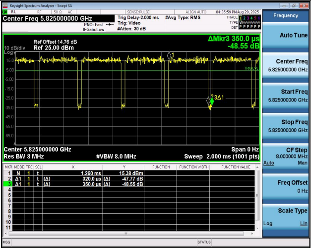
NTNV-11BE20MIMO-Ant1-5825
