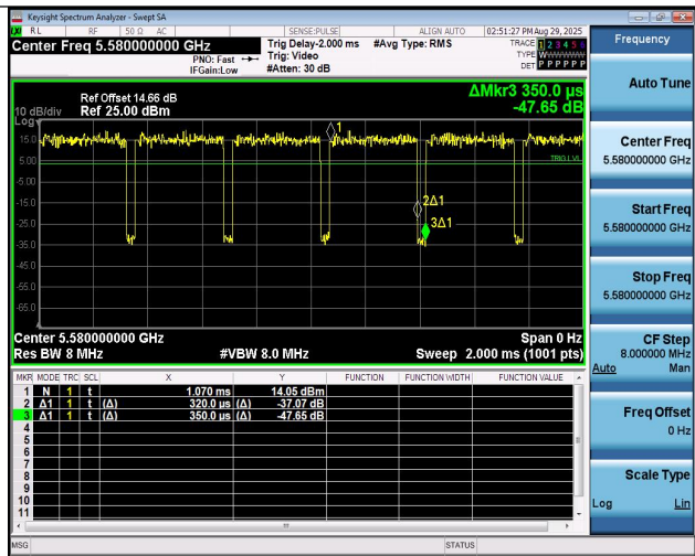
NTNV-11BE20MIMO-Ant1-5580
