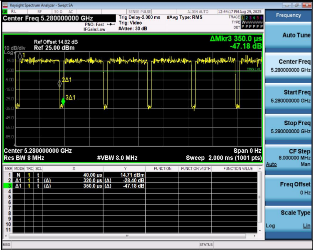
NTNV-11BE20MIMO-Ant2-5280
