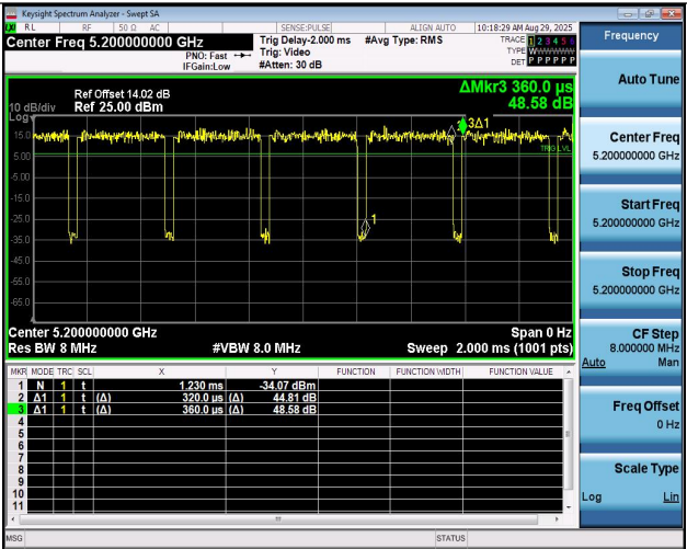
NTNV-11BE20MIMO-Ant1-5200
