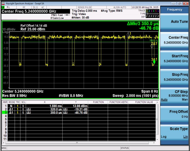
NTNV-11BE20MIMO-Ant1-5240
