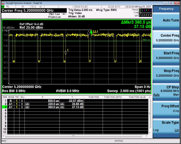
NTNV-11BE20MIMO-Ant2-5200
