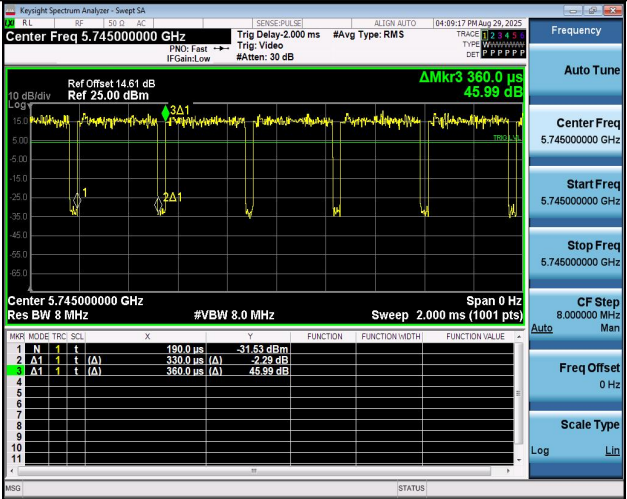
NTNV-11BE20MIMO-Ant1-5745
