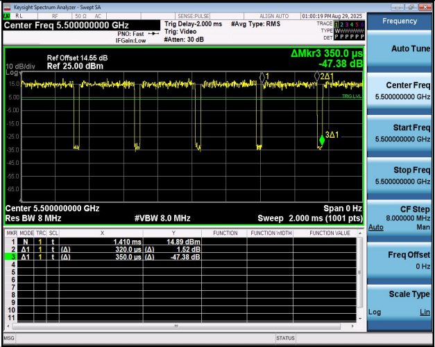
NTNV-11BE20MIMO-Ant1-5500
