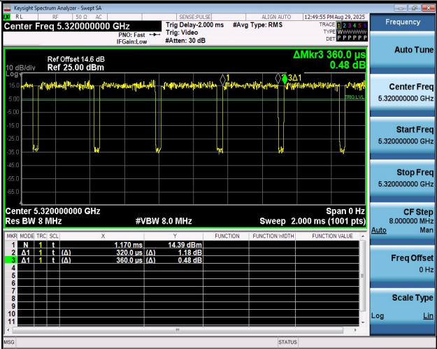
NTNV-11BE20MIMO-Ant1-5320
