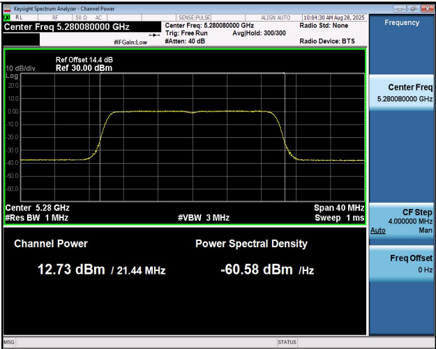
11AX20MIMO-Ant1-5280-PASS
