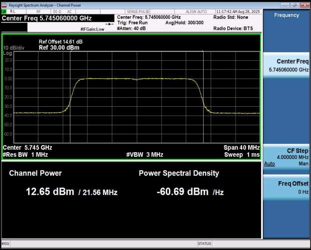
11AX20MIMO-Ant1-5745-PASS
