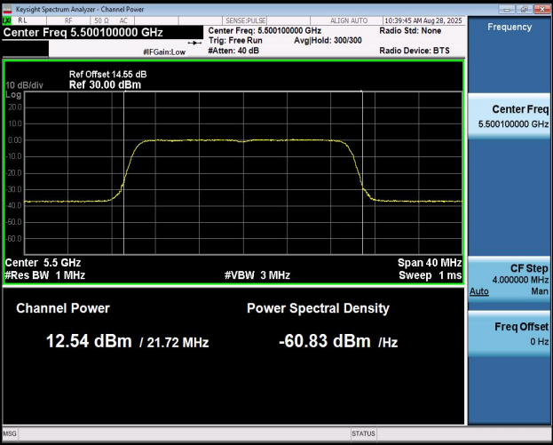
11AX20MIMO-Ant1-5500-PASS
