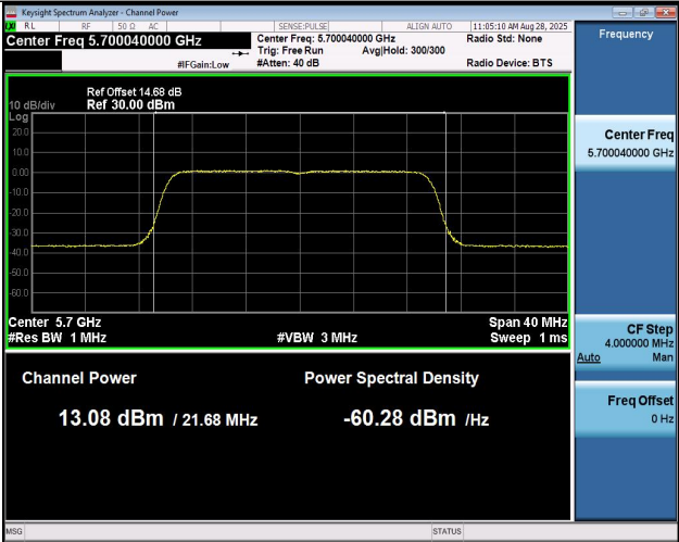
11AX20MIMO-Ant1-5700-PASS
