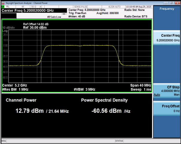
11BE20MIMO-Ant1-5200-PASS
