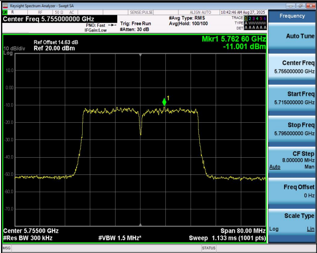
11N40MIMO-Ant1-5755-PASS
