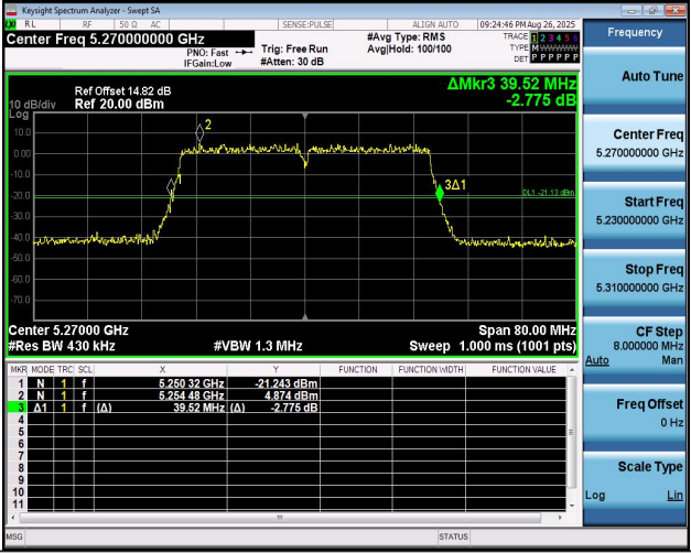
11N40MIMO-Ant2-5270
