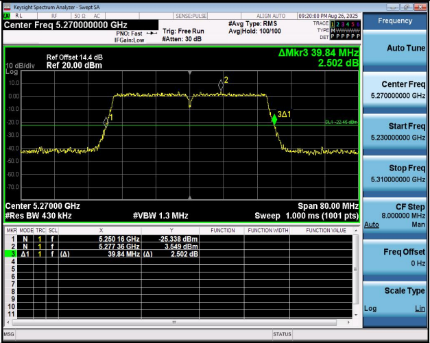
11N40MIMO-Ant1-5270
