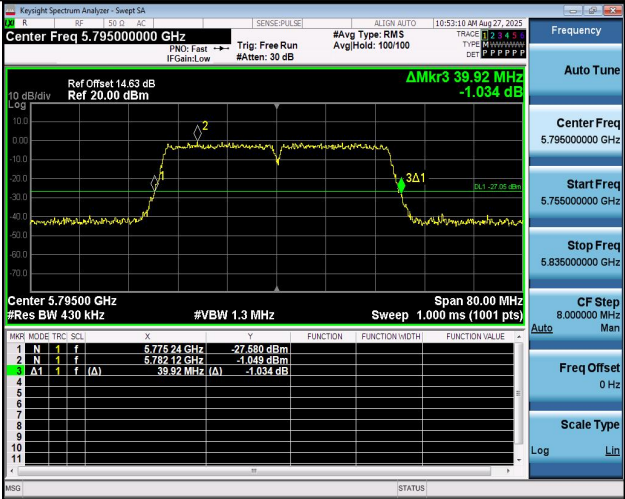
11N40MIMO-Ant1-5795
