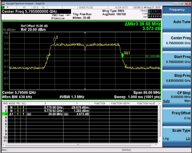
11N40MIMO-Ant2-5795
