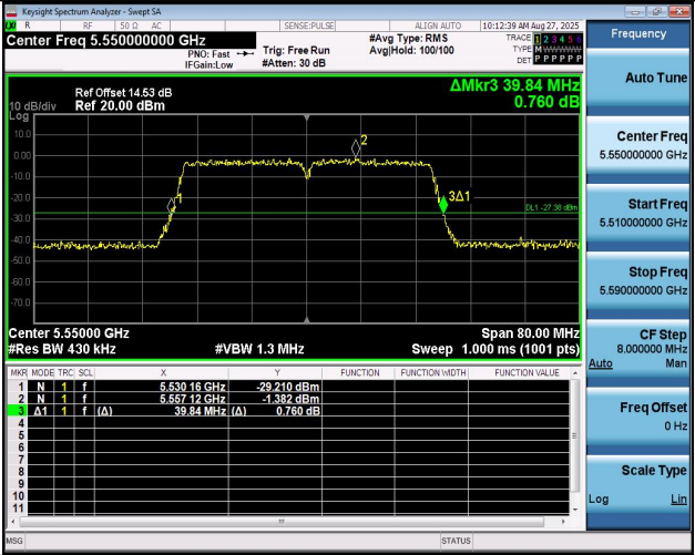
11N40MIMO-Ant1-5550
