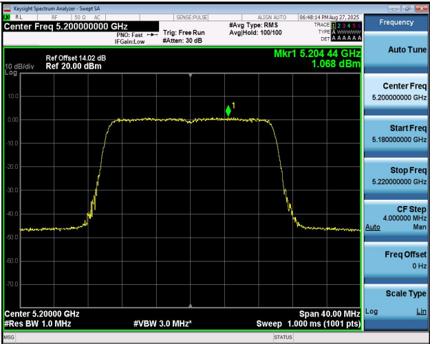
11AX20MIMO-Ant1-5200-PASS
