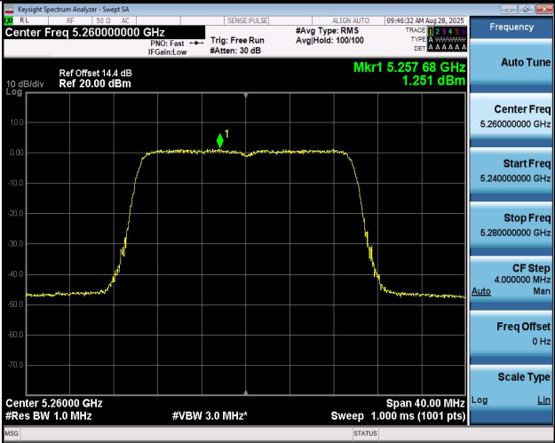
11AX20MIMO-Ant1-5260-PASS
