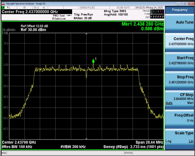
11AX20MIMO-Ant1-2437-PASS
