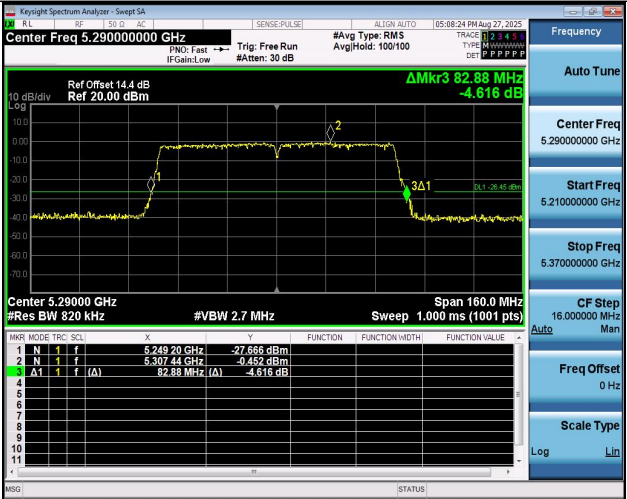
11AC80MIMO-Ant1-5290
