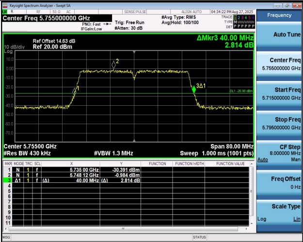
11AC40MIMO-Ant1-5755
