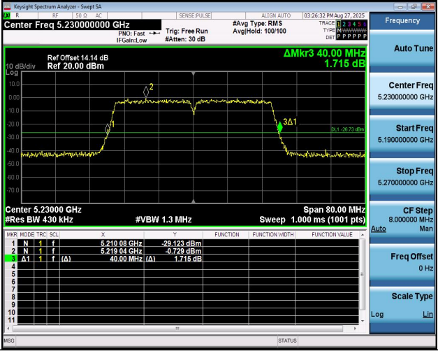
11AC40MIMO-Ant1-5230
