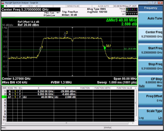
11AC40MIMO-Ant1-5270
