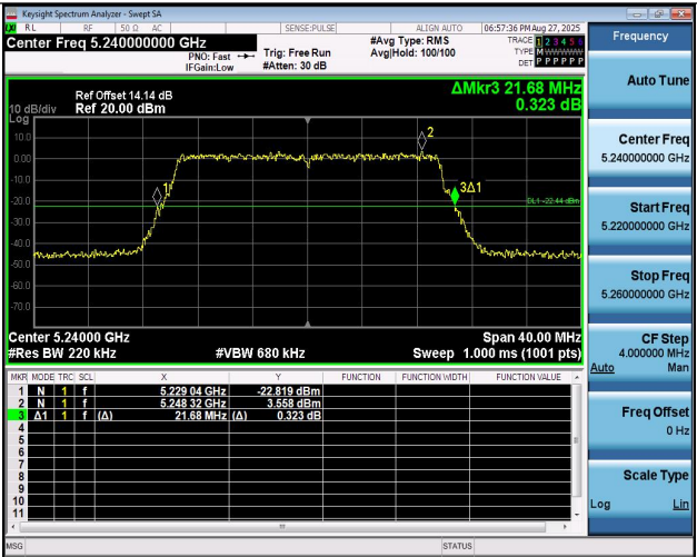
11AX20MIMO-Ant1-5240
