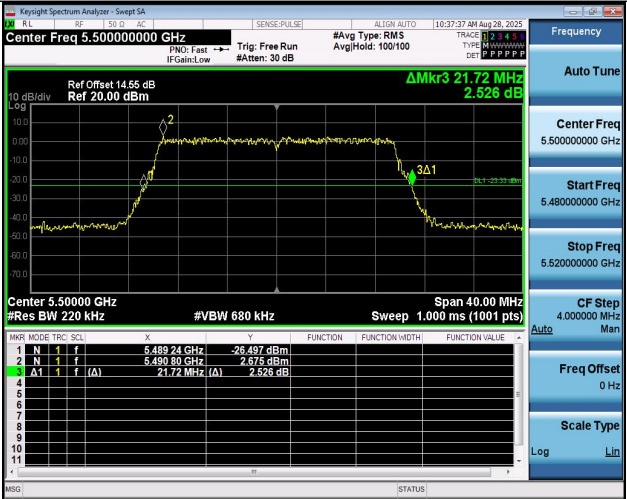
11AX20MIMO-Ant1-5500
