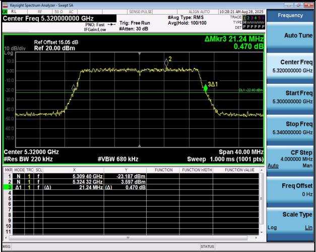
11AX20MIMO-Ant2-5320
