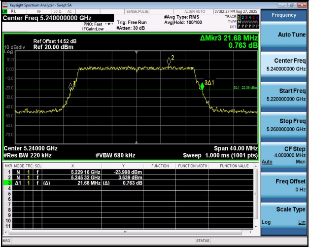
11AX20MIMO-Ant2-5240
