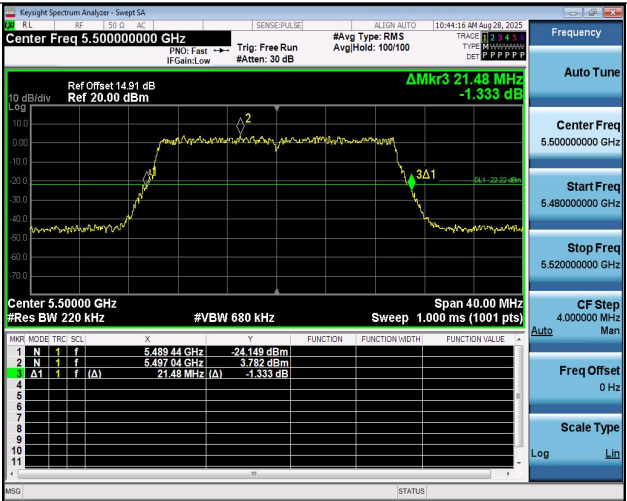
11AX20MIMO-Ant2-5500
