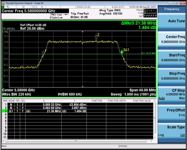
11AX20MIMO-Ant1-5580
