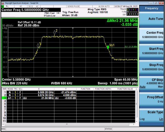
11AX20MIMO-Ant2-5580
