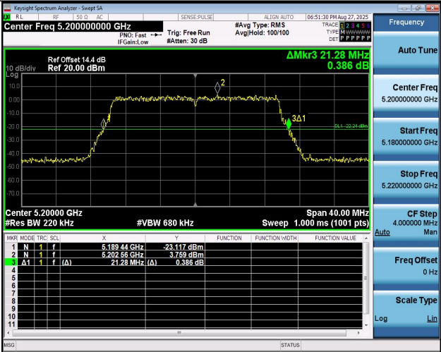
11AX20MIMO-Ant2-5200
