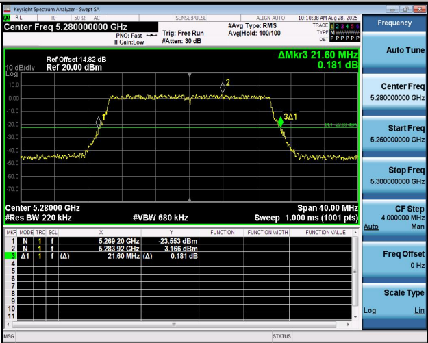
11AX20MIMO-Ant2-5280
