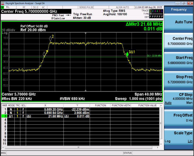
11AX20MIMO-Ant1-5700
