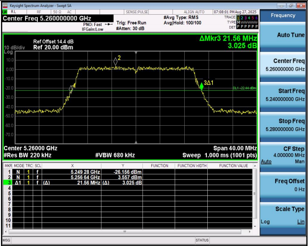
11AX20MIMO-Ant1-5260
