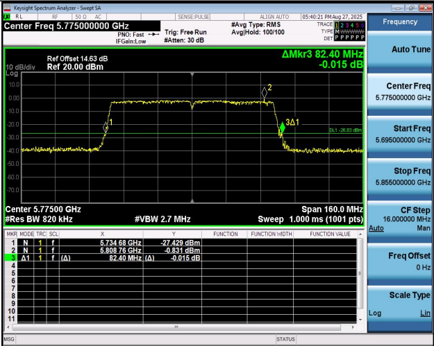
11AC80MIMO-Ant1-5775
