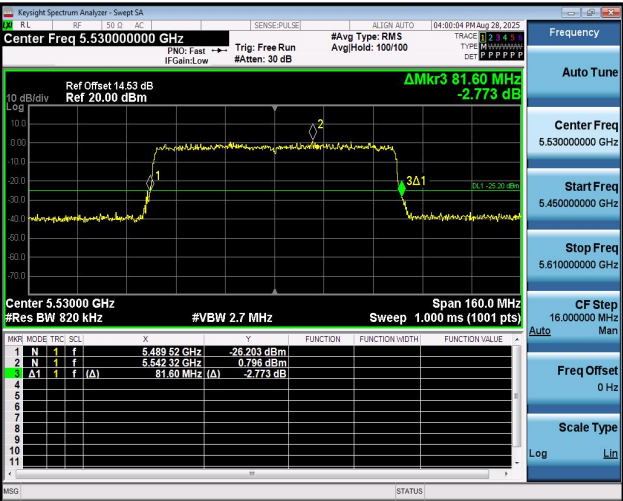
11AX80MIMO-Ant1-5530
