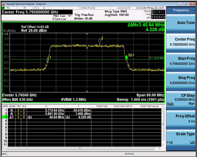
11AX40MIMO-Ant1-5795
