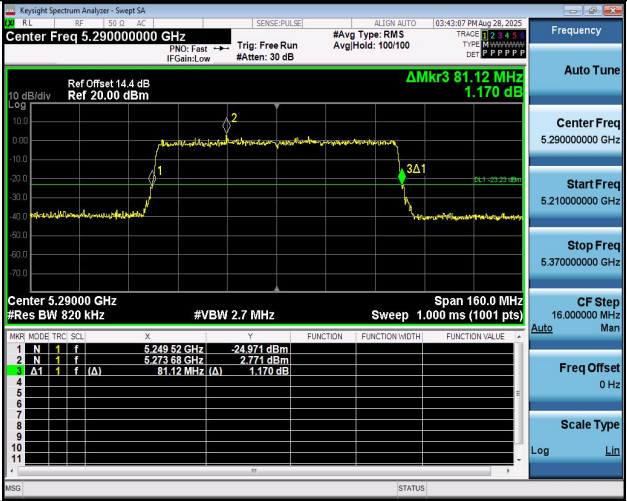
11AX80MIMO-Ant1-5290
