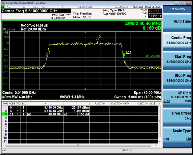
11AX40MIMO-Ant2-5510
