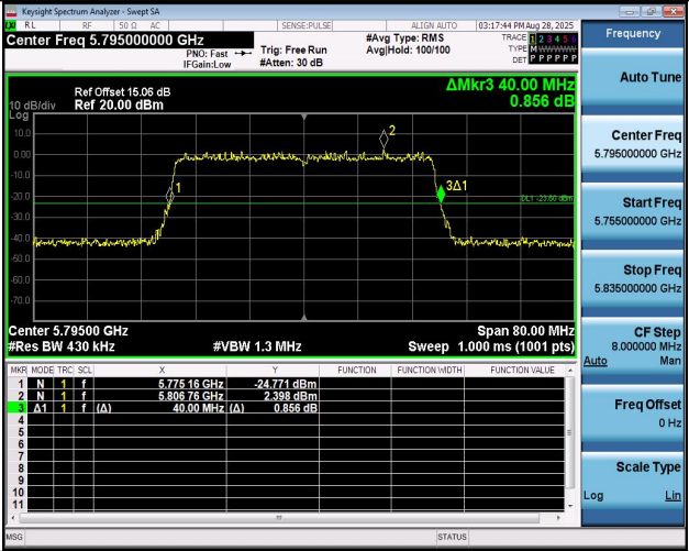
11AX40MIMO-Ant2-5795
