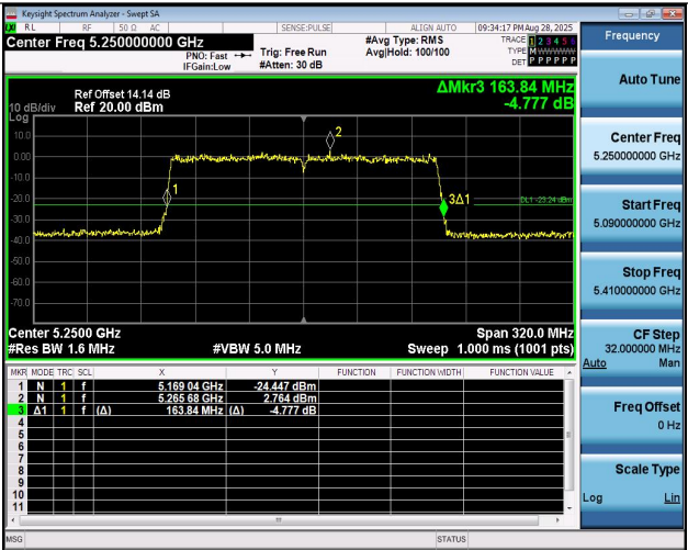
11AX160MIMO-Ant1-5250
