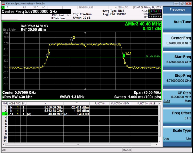
11AX40MIMO-Ant1-5670
