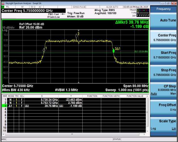
11AX40MIMO-Ant2-5755
