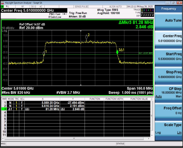
11AX80MIMO-Ant1-5610
