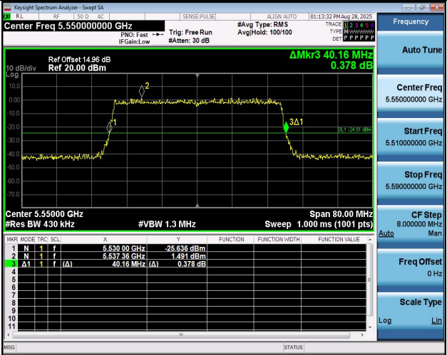
11AX40MIMO-Ant2-5550
