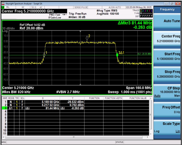
11AX80MIMO-Ant2-5210
