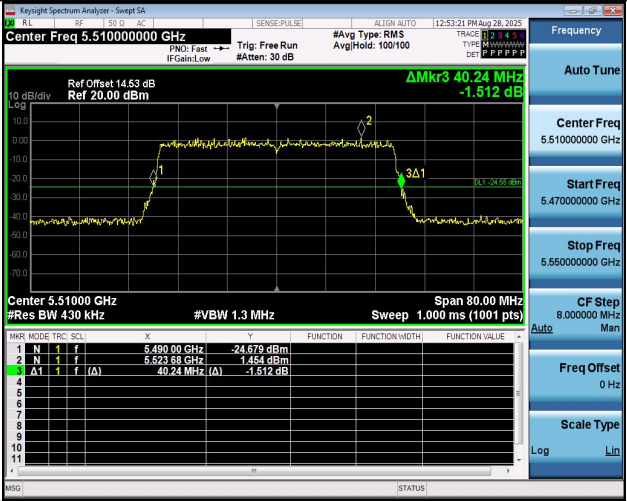
11AX40MIMO-Ant1-5510
