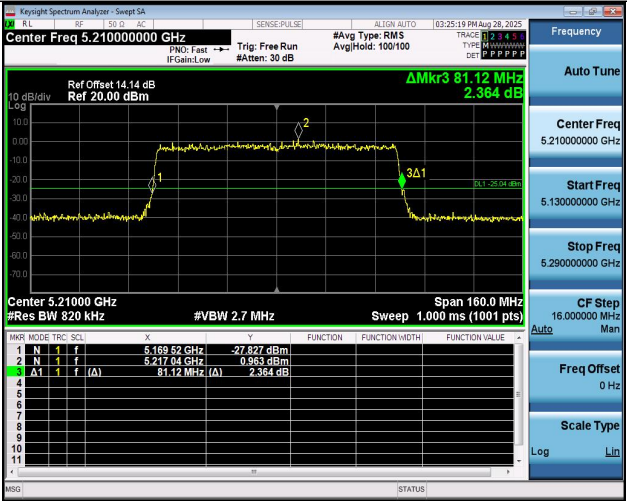
11AX80MIMO-Ant1-5210
