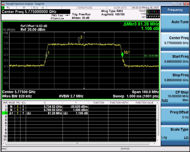
11AX80MIMO-Ant1-5775
