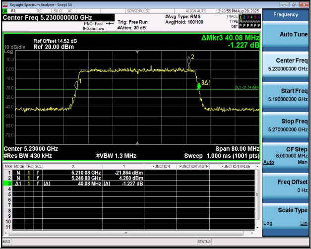
11AX40MIMO-Ant2-5230
