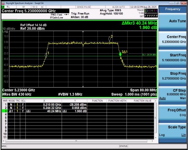
11AX40MIMO-Ant1-5230
