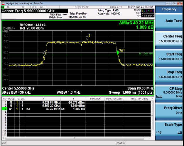
11BE40MIMO-Ant1-5550
