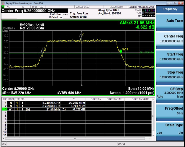
11BE20MIMO-Ant1-5260
