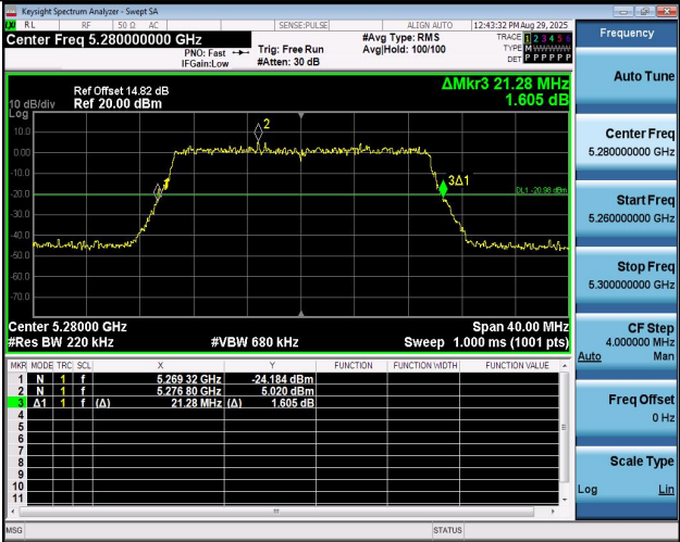
11BE20MIMO-Ant2-5280
