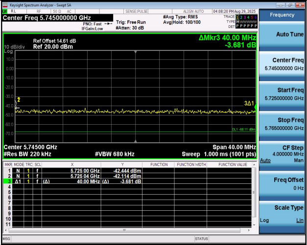
11BE20MIMO-Ant1-5745
