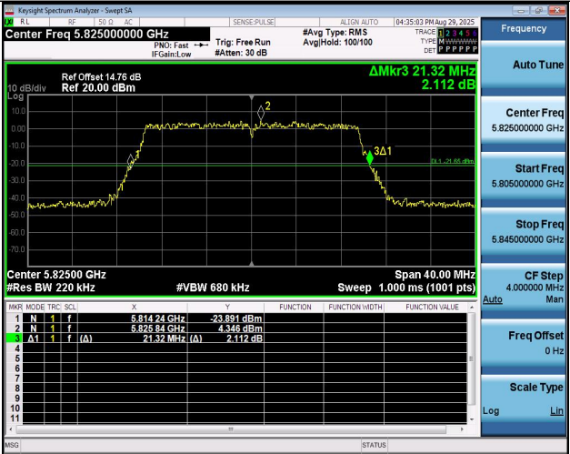
11BE20MIMO-Ant1-5825
