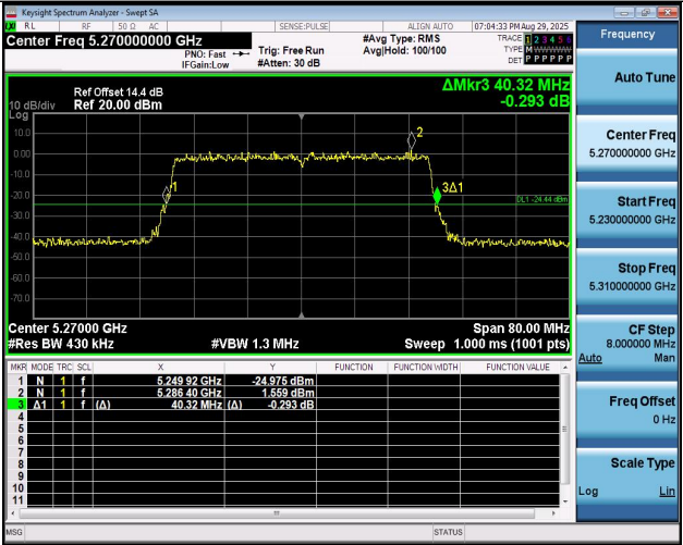
11BE40MIMO-Ant1-5270
