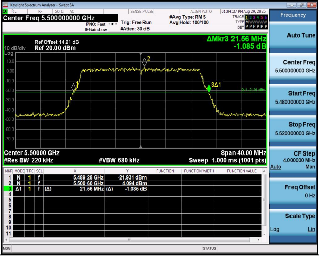
11BE20MIMO-Ant2-5500
