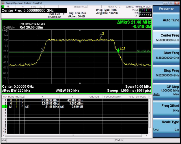
11BE20MIMO-Ant1-5500
