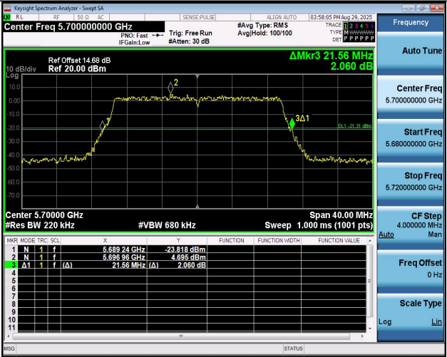
11BE20MIMO-Ant1-5700
