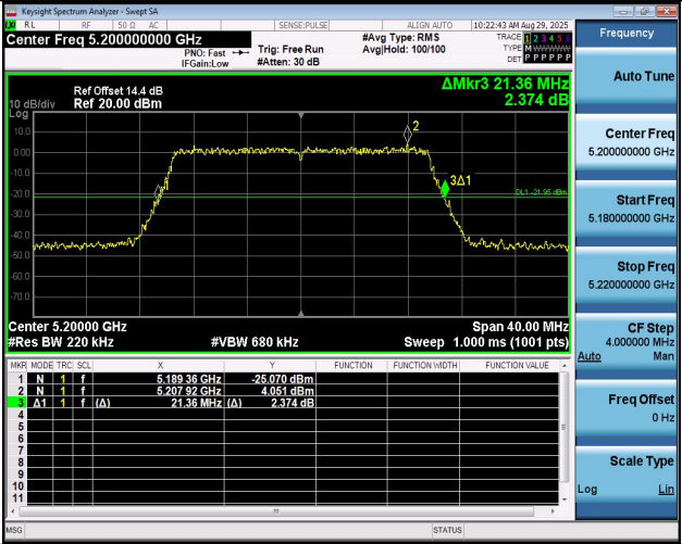
11BE20MIMO-Ant2-5200
