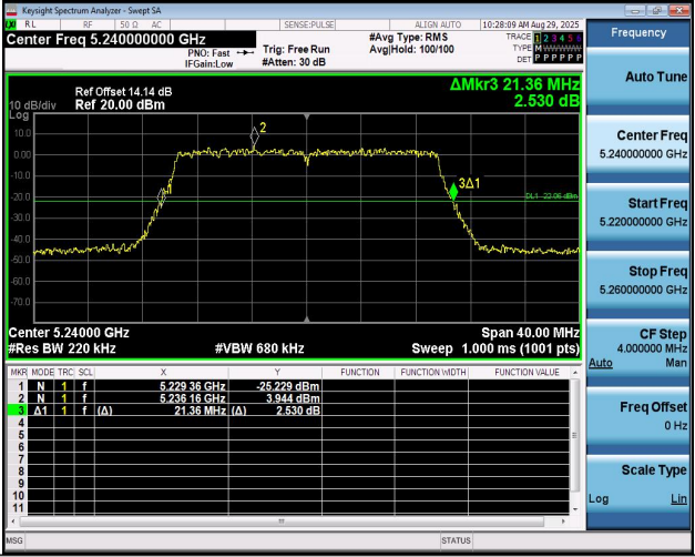
11BE20MIMO-Ant1-5240
