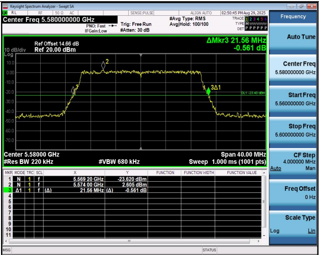
11BE20MIMO-Ant1-5580
