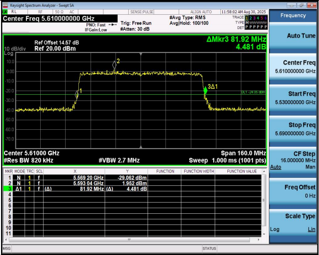
11BE80MIMO-Ant1-5610
