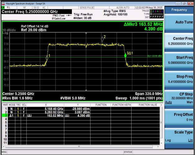
11BE160MIMO-Ant1-5250
