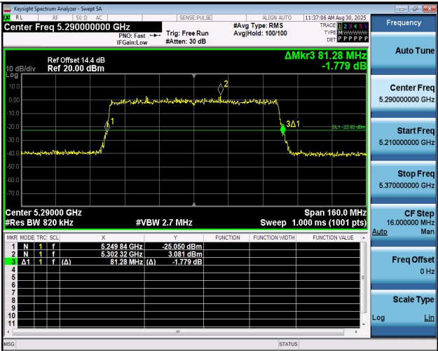
11BE80MIMO-Ant1-5290
