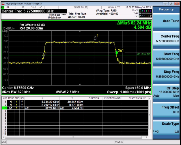
11BE80MIMO-Ant1-5775
