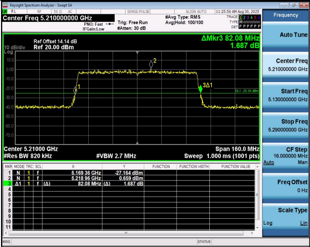
11BE80MIMO-Ant1-5210
