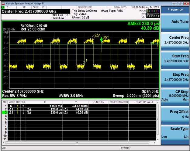
NTNV-11N40MIMO-Ant1-2437
