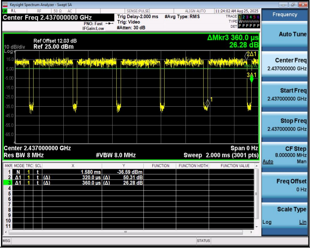
NTNV-11BE20MIMO-Ant1-2437
