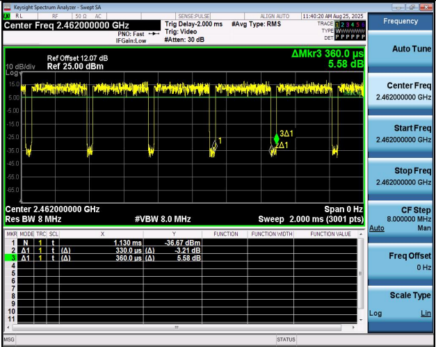
NTNV-11BE20MIMO-Ant1-2462
