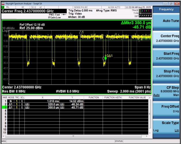
NTNV-11BE20MIMO-Ant2-2437
