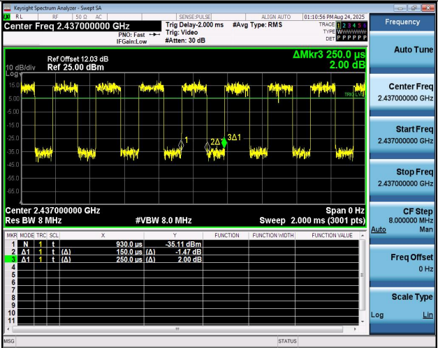
NTNV-11N20MIMO-Ant1-2437
