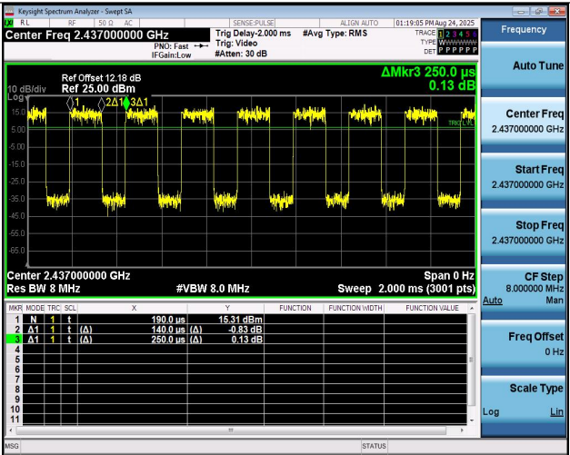
NTNV-11N20MIMO-Ant2-2437
