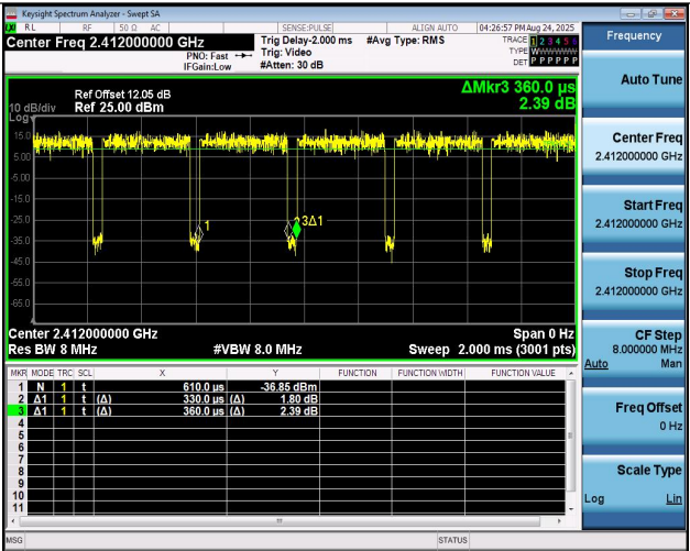
NTNV-11AX20MIMO-Ant1-2412
