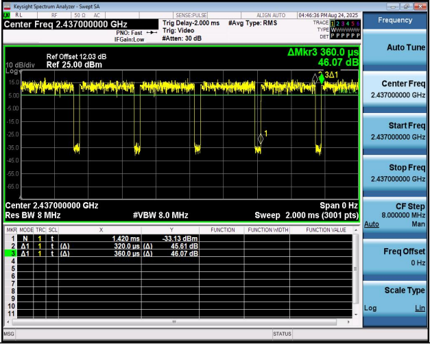
NTNV-11AX20MIMO-Ant1-2437
