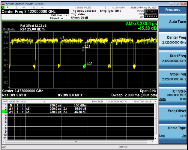
NTNV-11AX40MIMO-Ant1-2422
