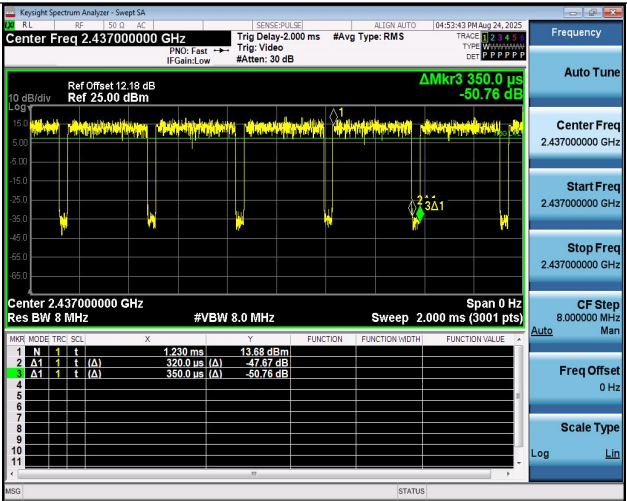
NTNV-11AX20MIMO-Ant2-2437
