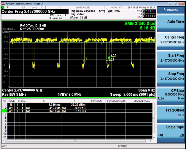
NTNV-11AX40MIMO-Ant2-2437
