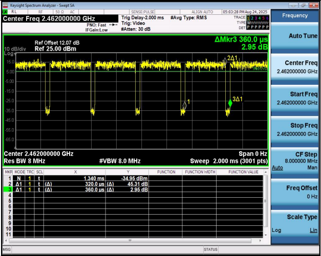
NTNV-11AX20MIMO-Ant1-2462
