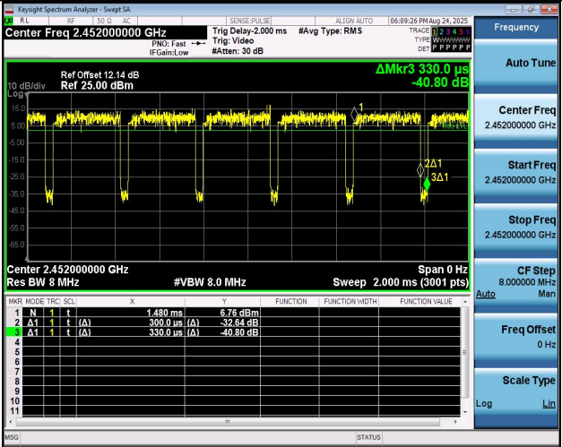
NTNV-11AX40MIMO-Ant1-2452
