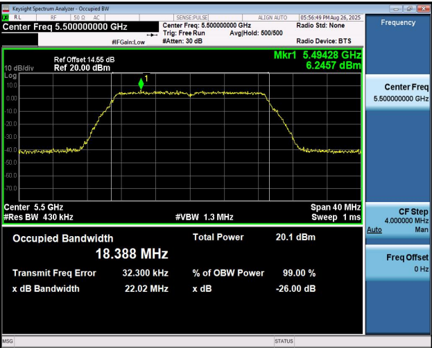
11N20MIMO-Ant1-5500
