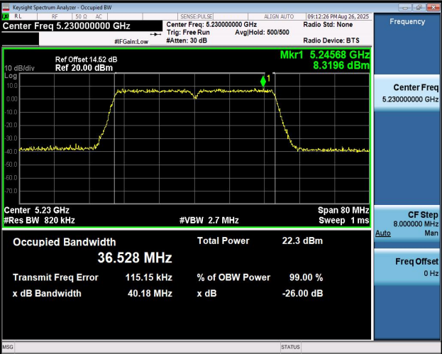
11N40MIMO-Ant2-5230
