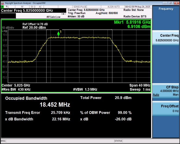
11N20MIMO-Ant1-5825
