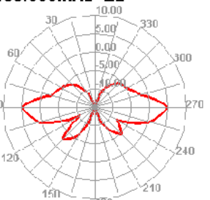
5150.000MHz E2
