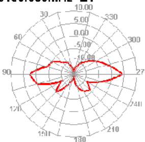
5150.000MHz E1
