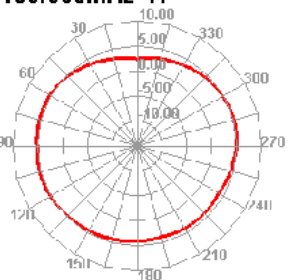
5150.000MHz H
