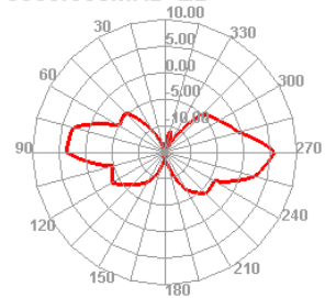
5500.000MHz E2
