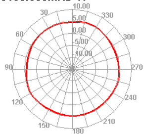
5150.000MHz H
