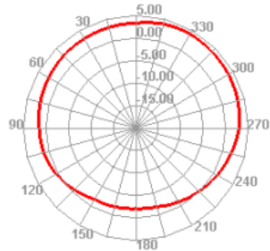
5150.000MHz H
