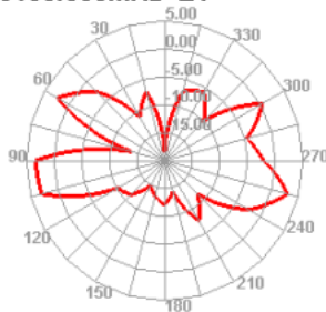
5150.000MHz E1
