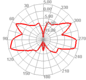
5150.000MHz E2
