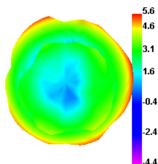
5500.000MHz E1
