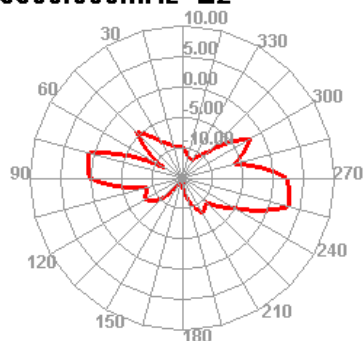
5500.000MHz E2
