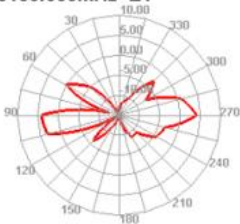
5500.000MHz E1
