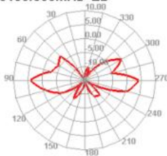
5500.000MHz E2
