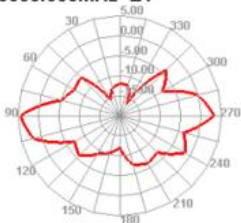
5850.000MHz E1
