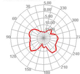
5500.000MHz E2
