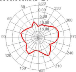
5500.000MHz E1
