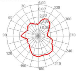
5850.000MHz H
