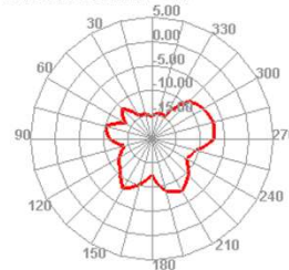
5500.000MHz E1
