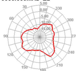
5500.000MHz E2
