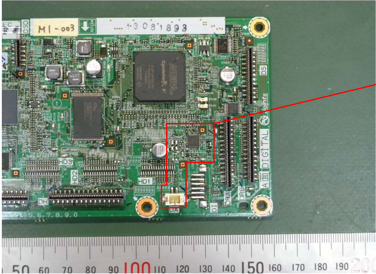
RFID Module
