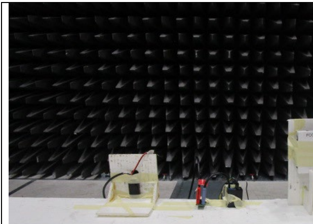
EUT Orientation
