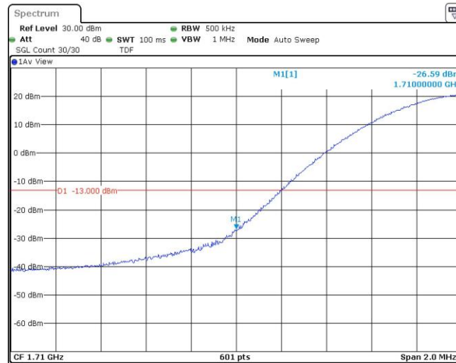
Band4-20MHz-QPSK-20050-1RB#99
