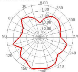
2450.000MHz H
