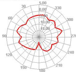
2450.000MHz E2
