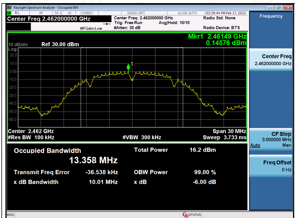
Test_Graph_802.11b_ANT1_2462_1Mbps_DTSSBW
