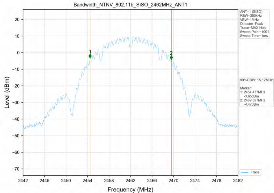
802.11b_2462MHz_SISO_ANT1
