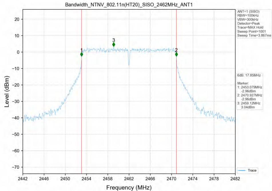
802.11n(HT20)_2462MHz_SISO_ANT1
