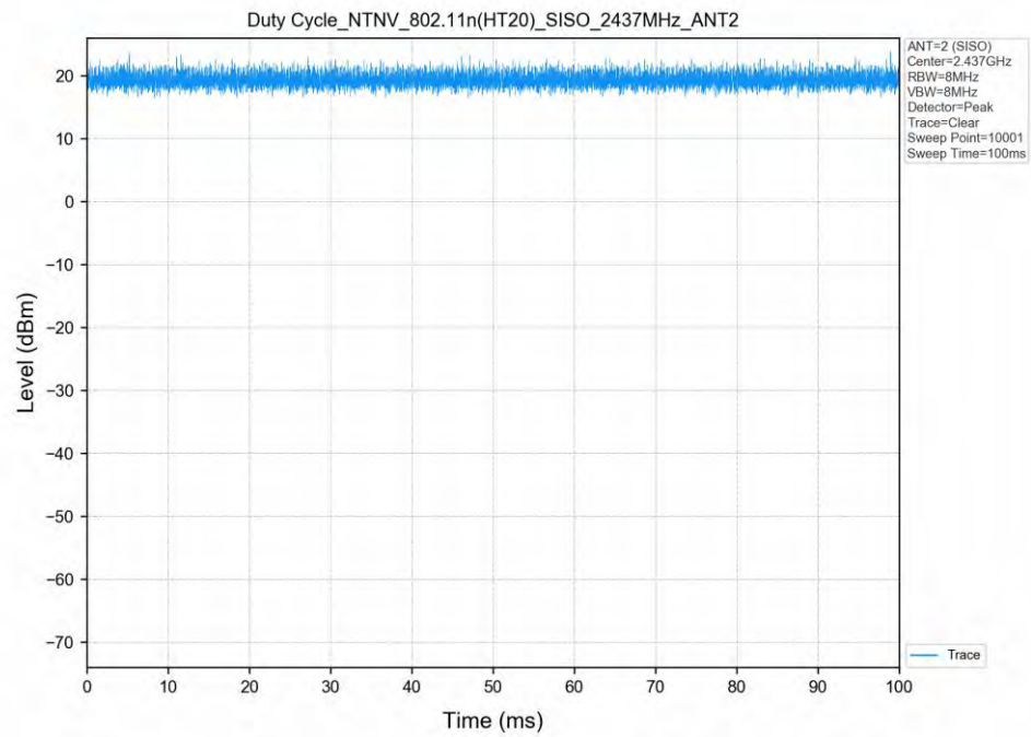
802.11n(HT20)_2437MHz_SISO_ANT2
