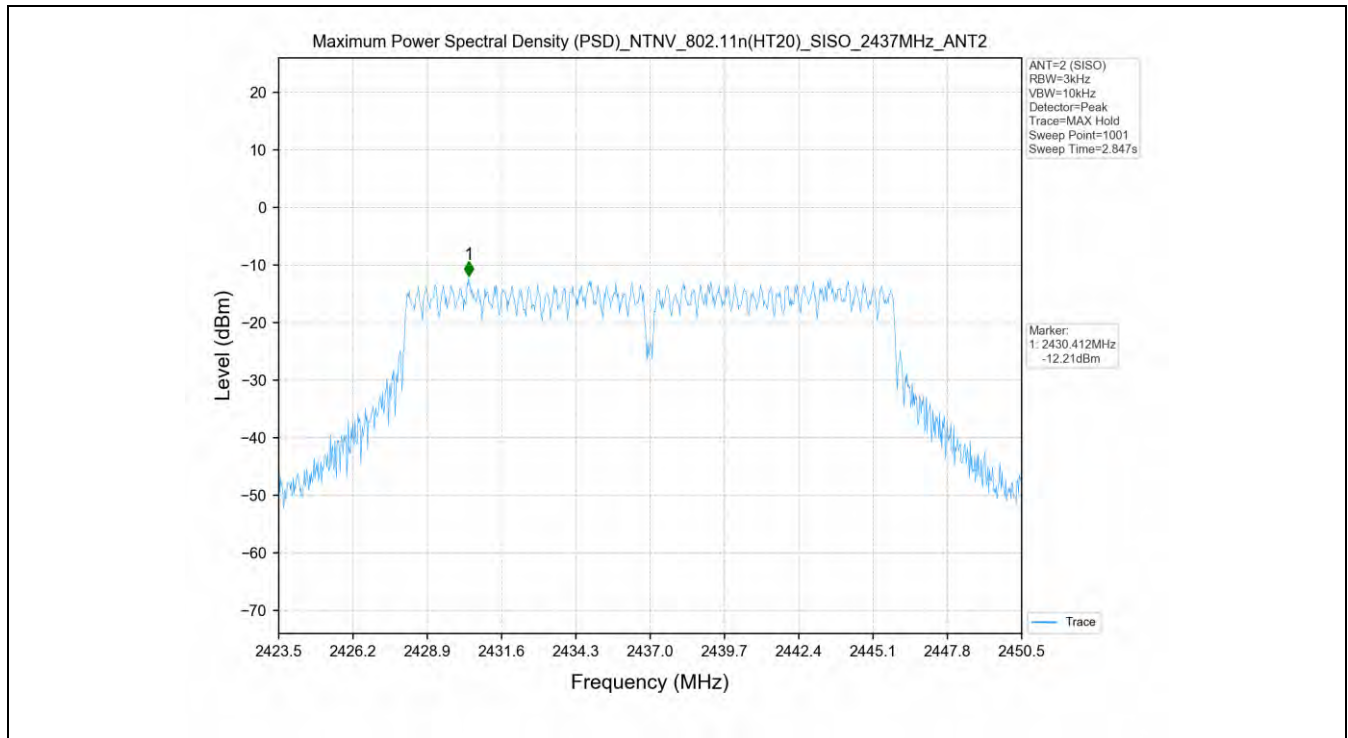
802.11n(HT20)_2437MHz_SISO_ANT2
