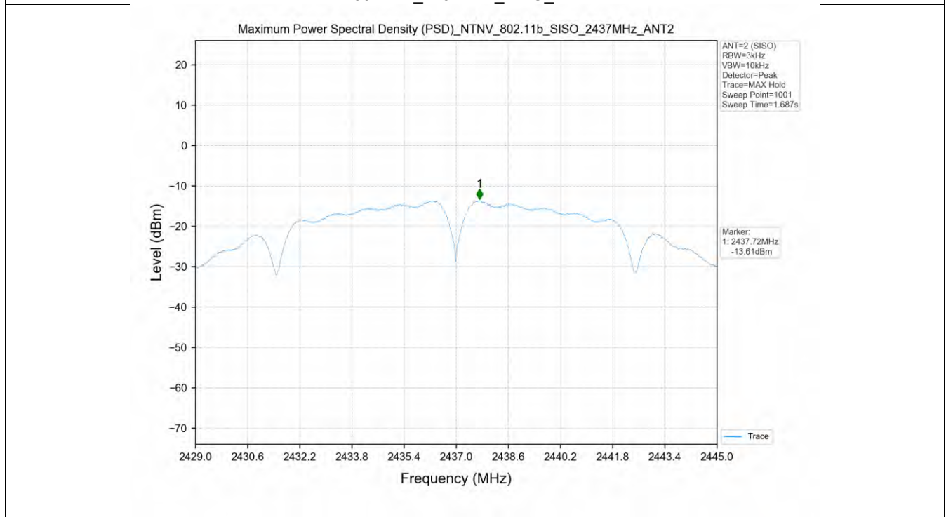
802.11b_2437MHz_SISO_ANT2
