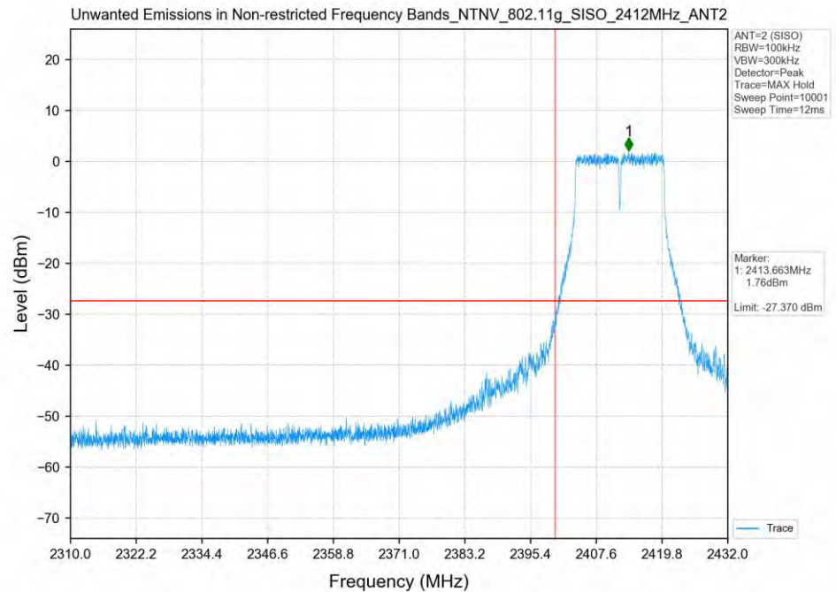
802.11g_2412MHz_SISO_ANT2
