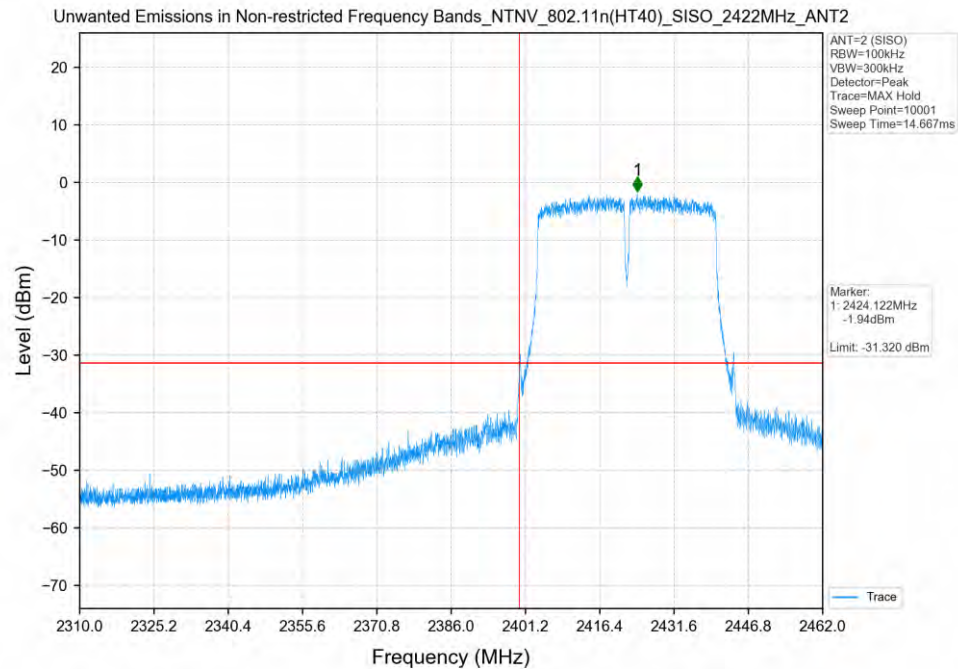
802.11n(HT40)_2422MHz_SISO_ANT2
