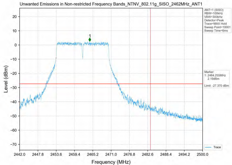
802.11g_2462MHz_SISO_ANT1
