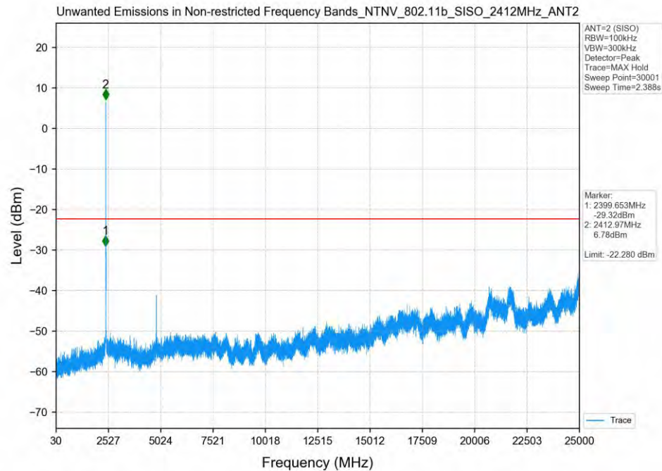
802.11b_2412MHz_SISO_ANT2
