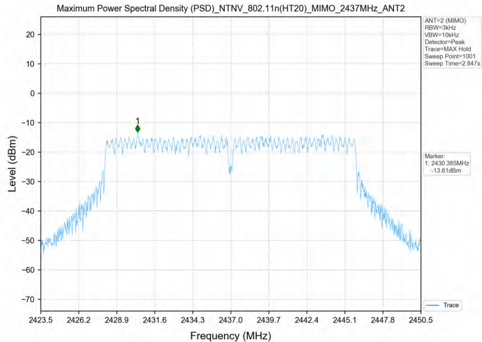
802.11n(HT20)_2437MHz_MIMO_ANT2
