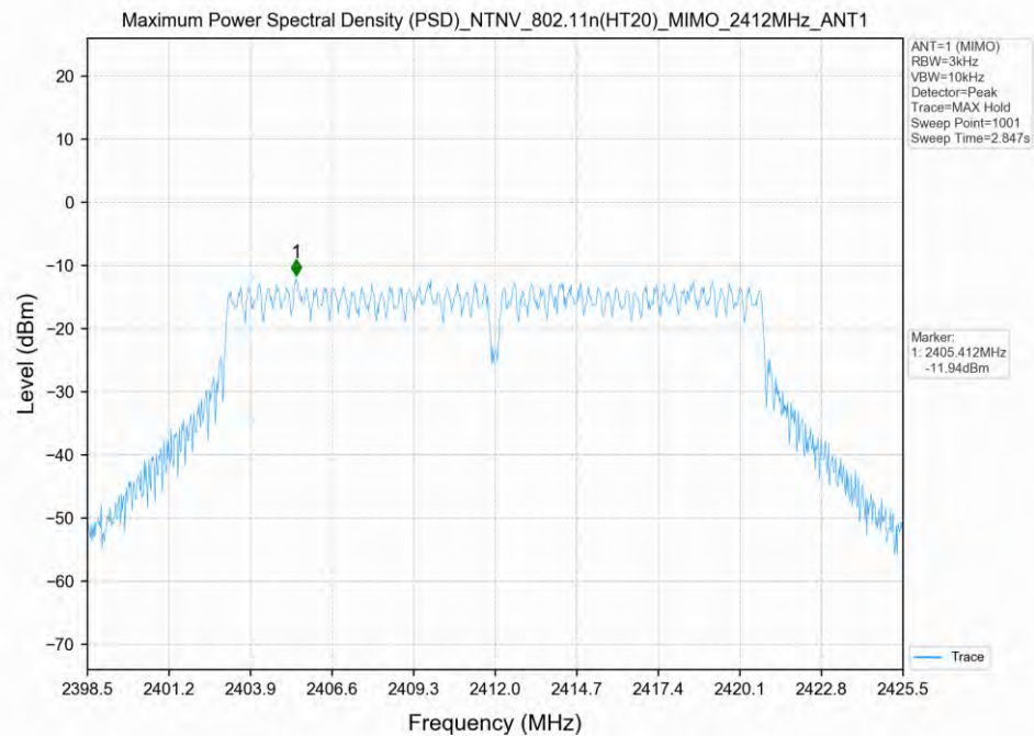
802.11n(HT20)_2412MHz_MIMO_ANT1
