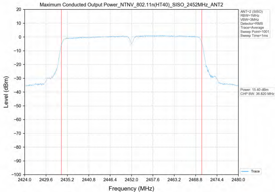
802.11n(HT40)_2452MHz_SISO_ANT2
