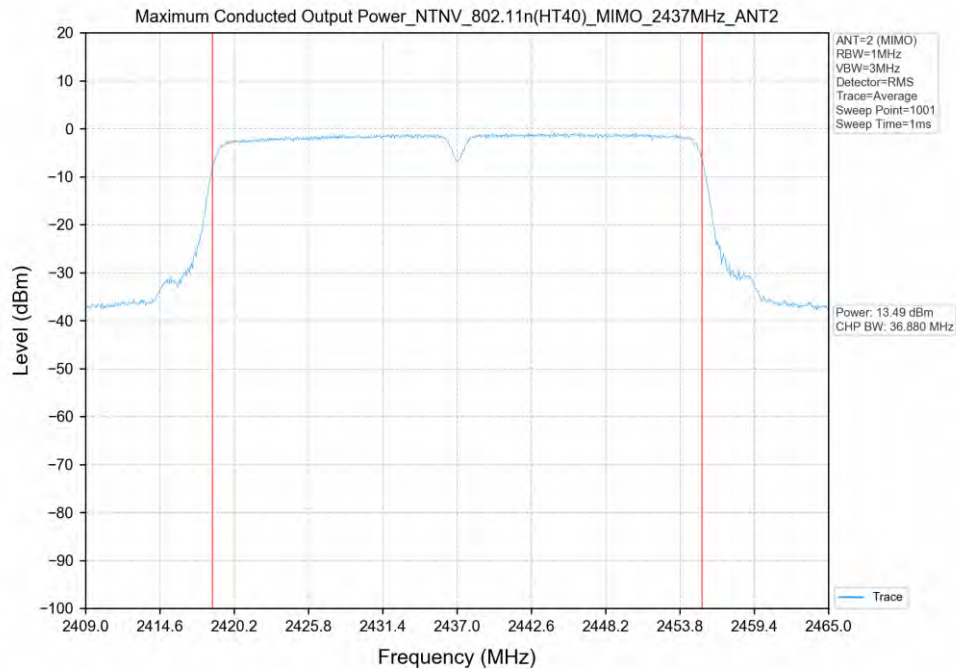
802.11n(HT40)_2437MHz_MIMO_ANT2
