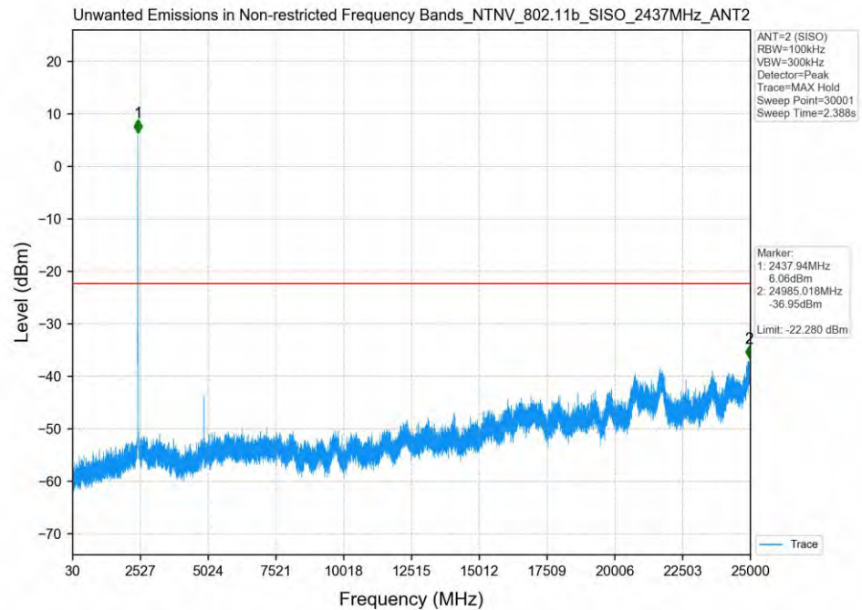
802.11b_2437MHz_SISO_ANT2
