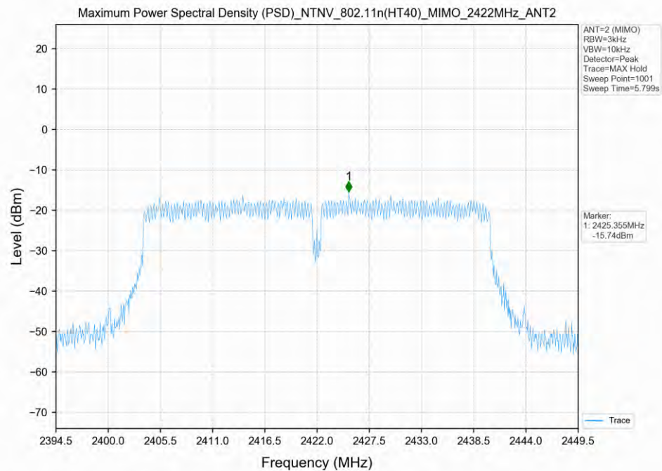
802.11n(HT40)_2422MHz_MIMO_ANT2
