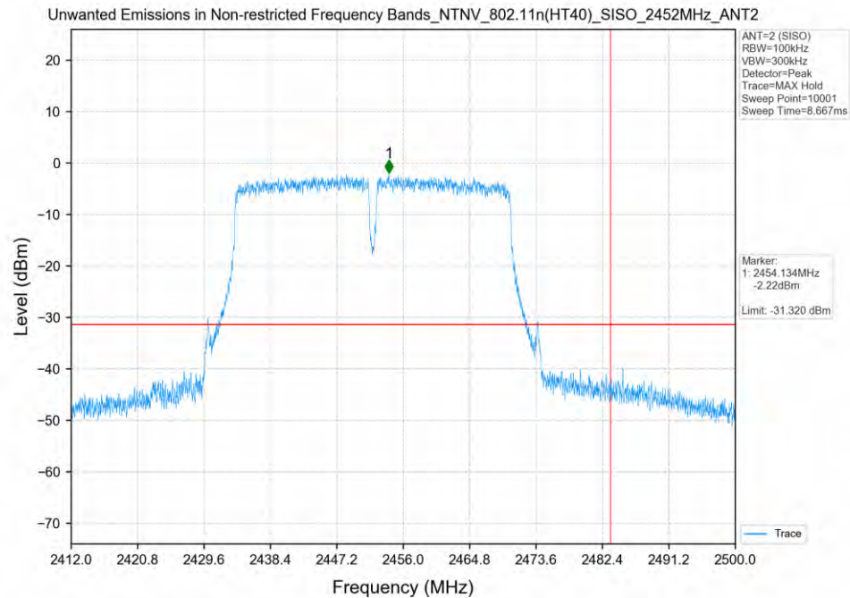
802.11n(HT40)_2452MHz_SISO_ANT2
