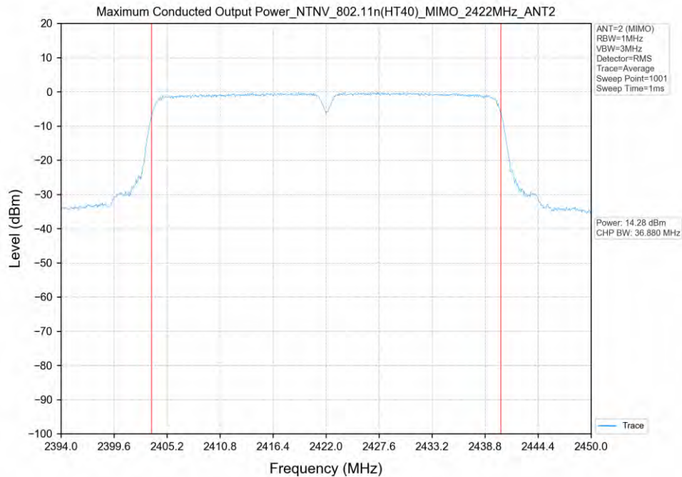
802.11n(HT40)_2422MHz_MIMO_ANT2
