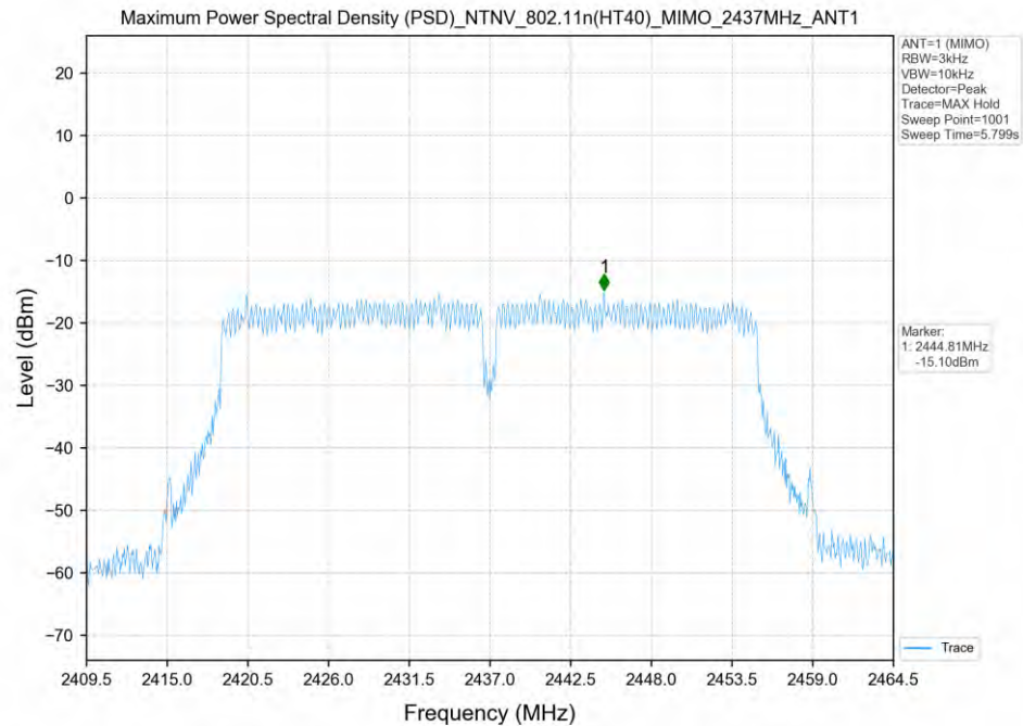
802.11n(HT40)_2437MHz_MIMO_ANT1
