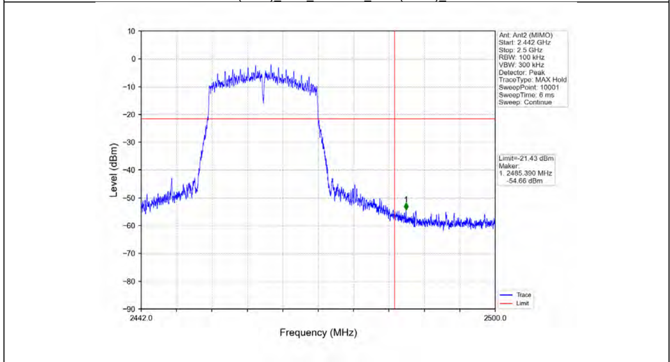
802.11n(HT20)_HCH_2462MHz_Ant2 (MIMO)_NTNV
