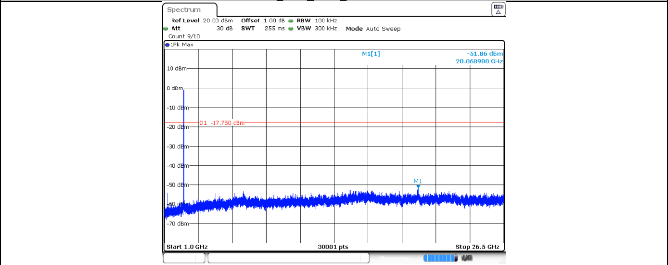
11B_Ant1_2462_0~Reference
