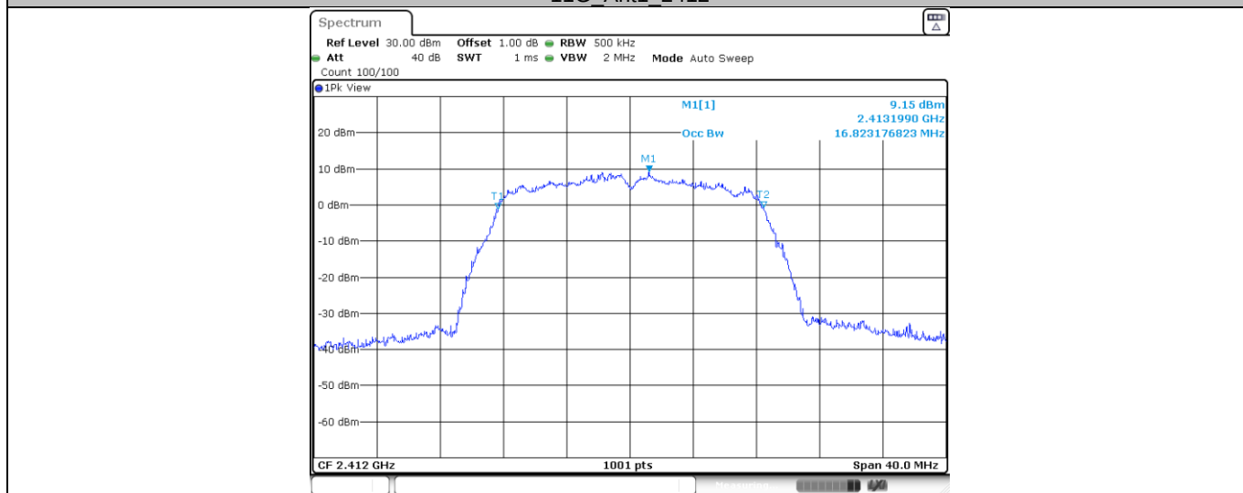
11G Ant1 2412
