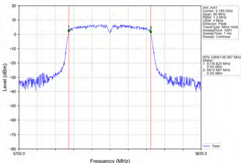
802.11n(HT40)_HCH_5795MHz_Ant1_NTNV
