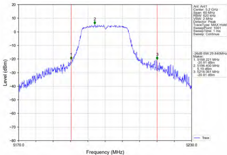
802.11a_MCH_5200MHz_Ant1_NTNV
