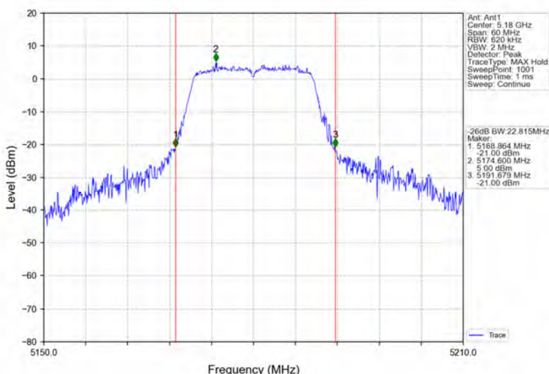
802.11n(HT20)_LCH_5180MHz_Ant1_NTNV
