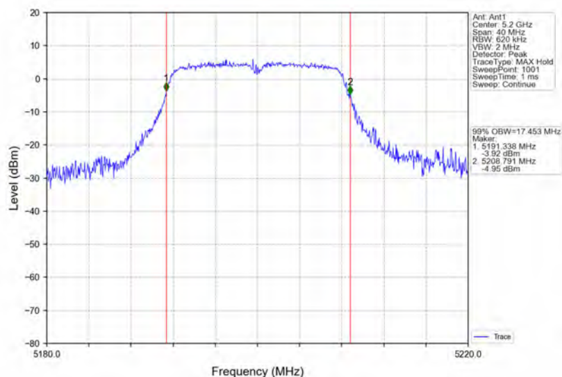
802.11a_MCH_5200MHz_Ant1_NTNV
