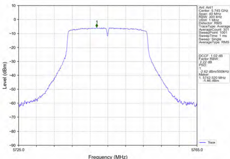
802.11n(HT20)_LCH_5745MHz_Ant1_NTNV
