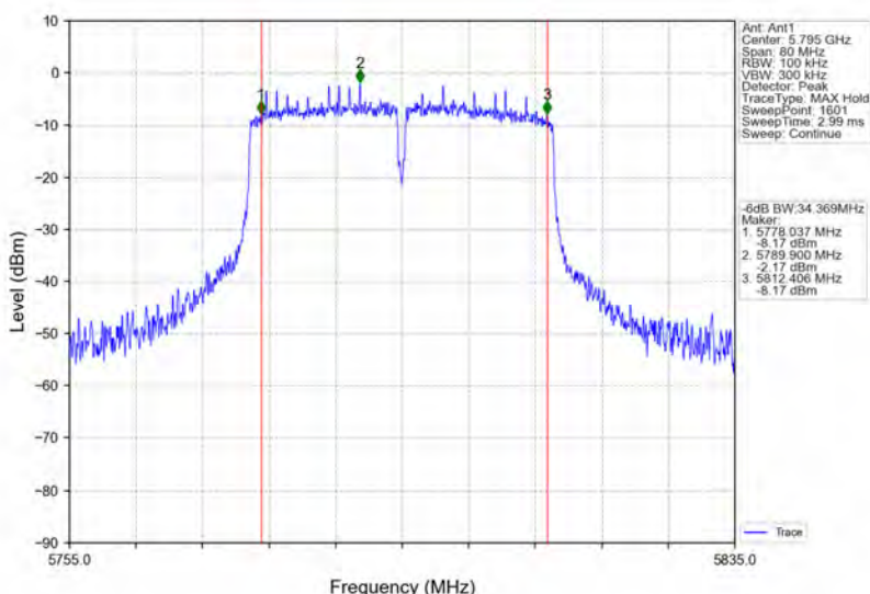
802.11n(HT40)_HCH_5795MHz_Ant1_NTNV
