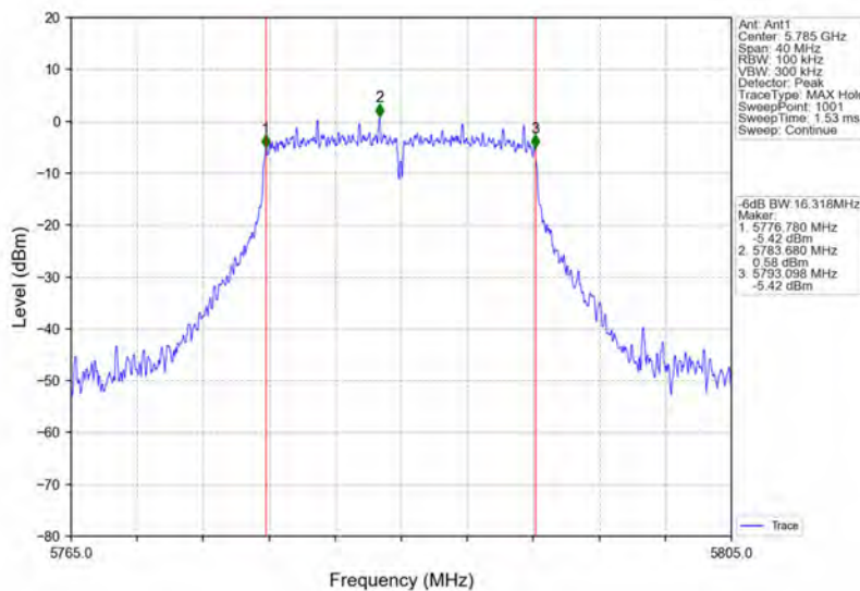
802.11a_MCH_5785MHz_Ant1_NTNV
