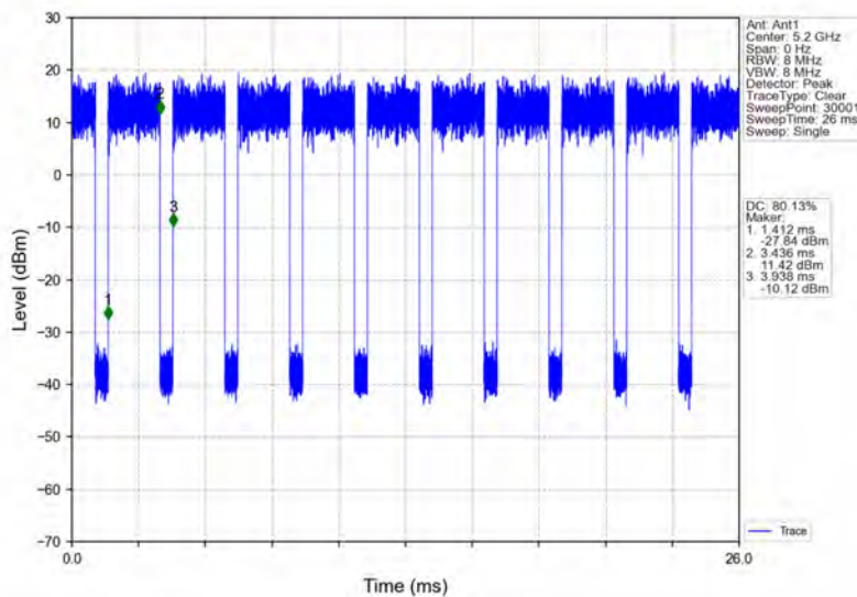
802.11a_MCH_5200MHz_Ant1_NTNV
