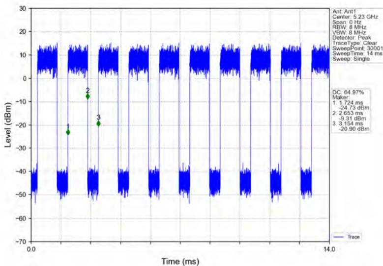
802.11n(HT40)_HCH_5230MHz_Ant1_NTNV
