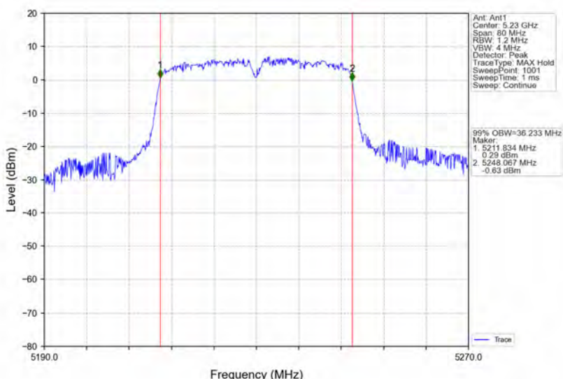
802.11n(HT40)_HCH_5230MHz_Ant1_NTNV
