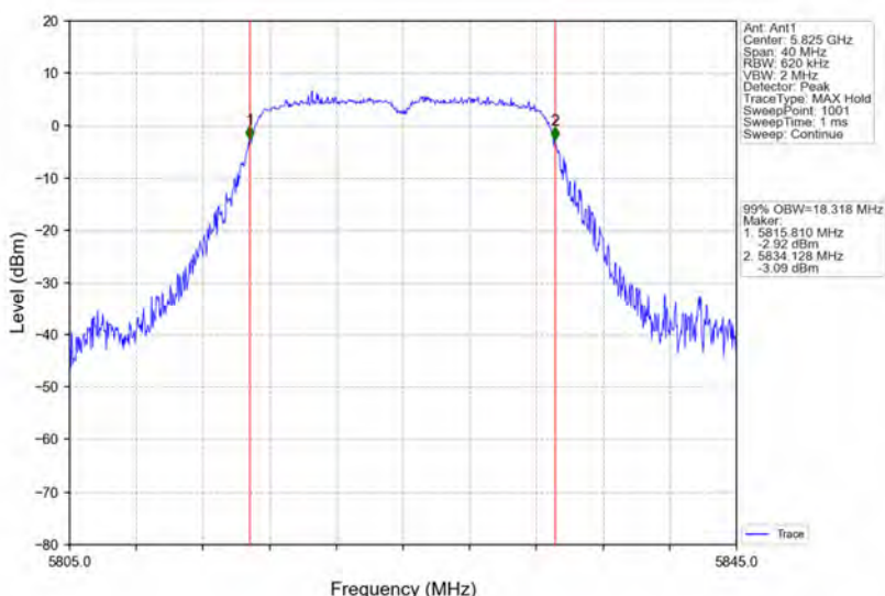
802.11n(HT20)_HCH_5825MHz_Ant1_NTNV
