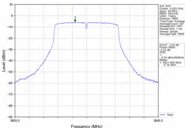
802.11n(HT20)_HCH_5825MHz_Ant1_NTNV
