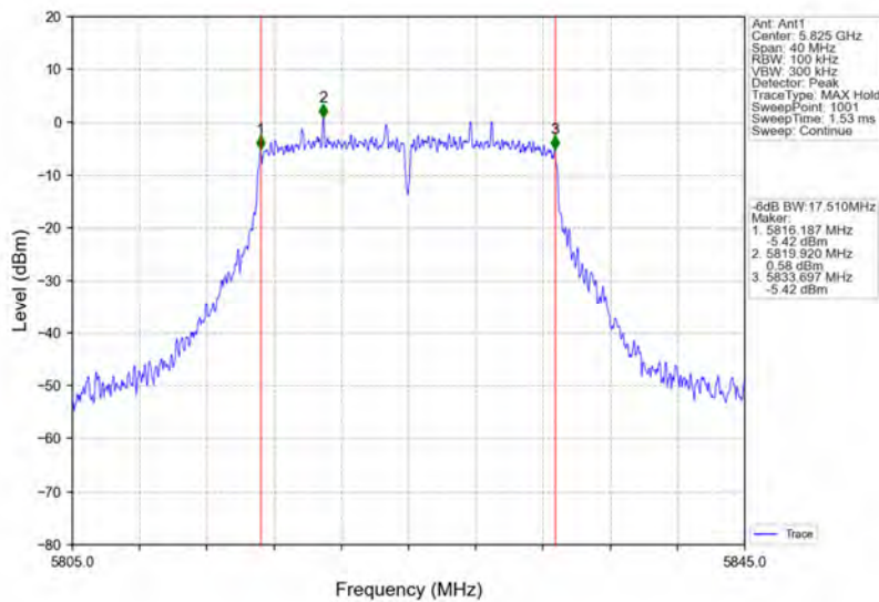
802.11n(HT20)_HCH_5825MHz_Ant1_NTNV
