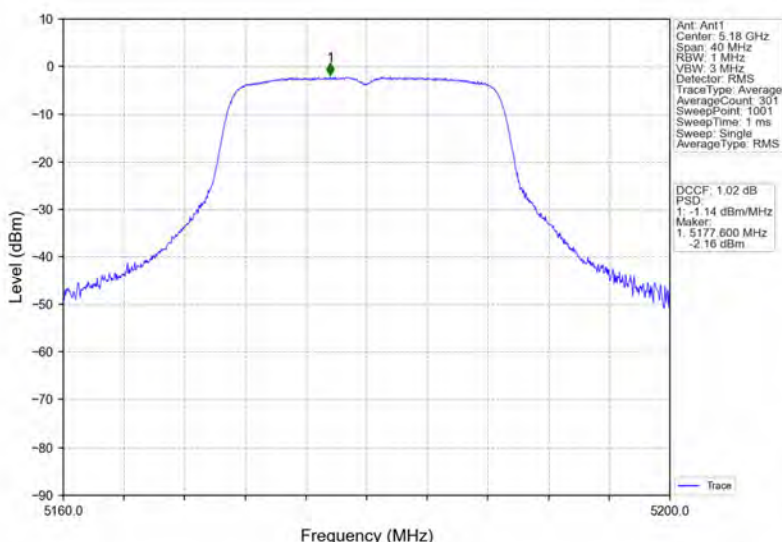
802.11n(HT20)_LCH_5180MHz_Ant1_NTNV
