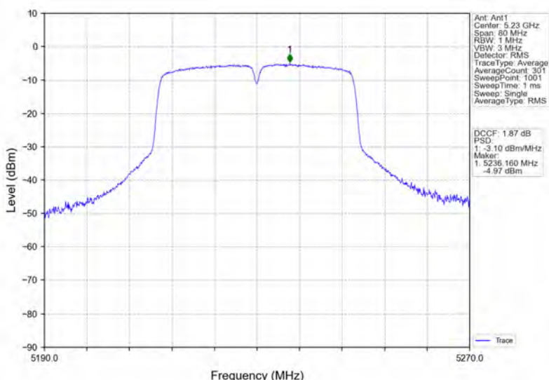
802.11n(HT40)_HCH_5230MHz_Ant1_NTNV
