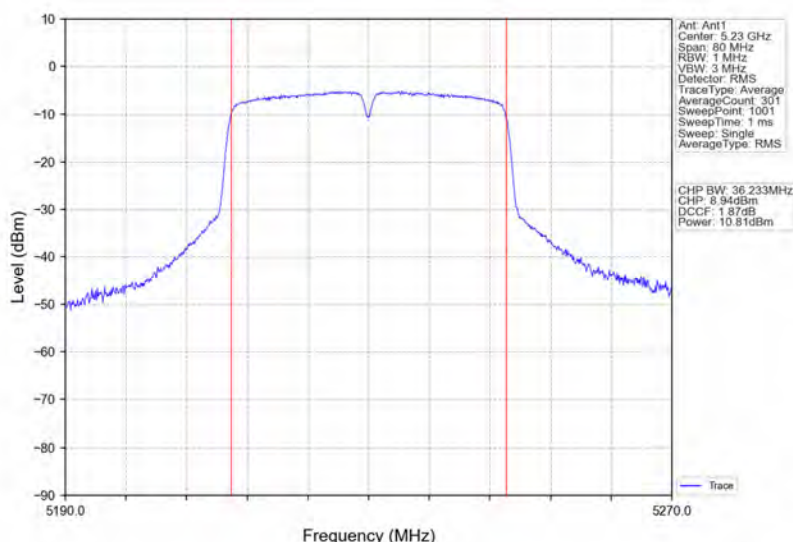
802.11n(HT40)_HCH_5230MHz_Ant1_NTNV
