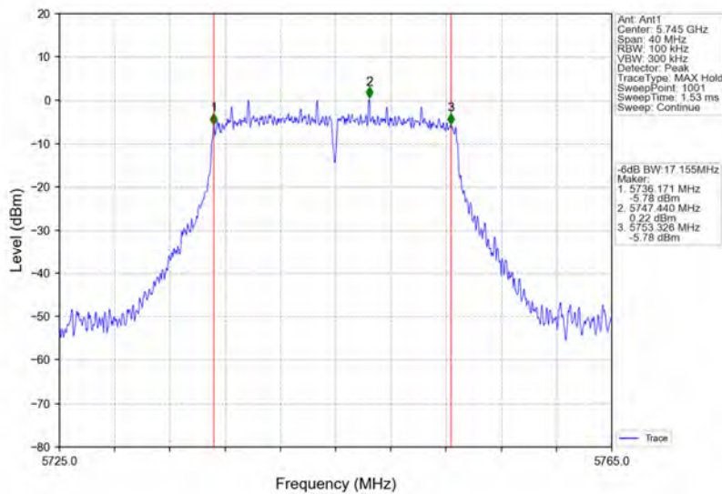
802.11n(HT20)_LCH_5745MHz_Ant1_NTNV
