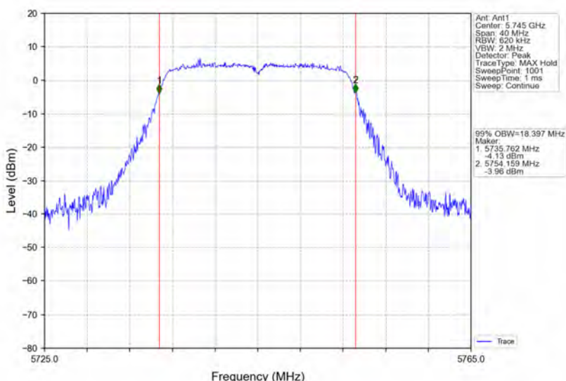
802.11n(HT20)_LCH_5745MHz_Ant1_NTNV
