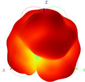
5500.0MHz Total(E1-XZ), Max= 1.30dBi
