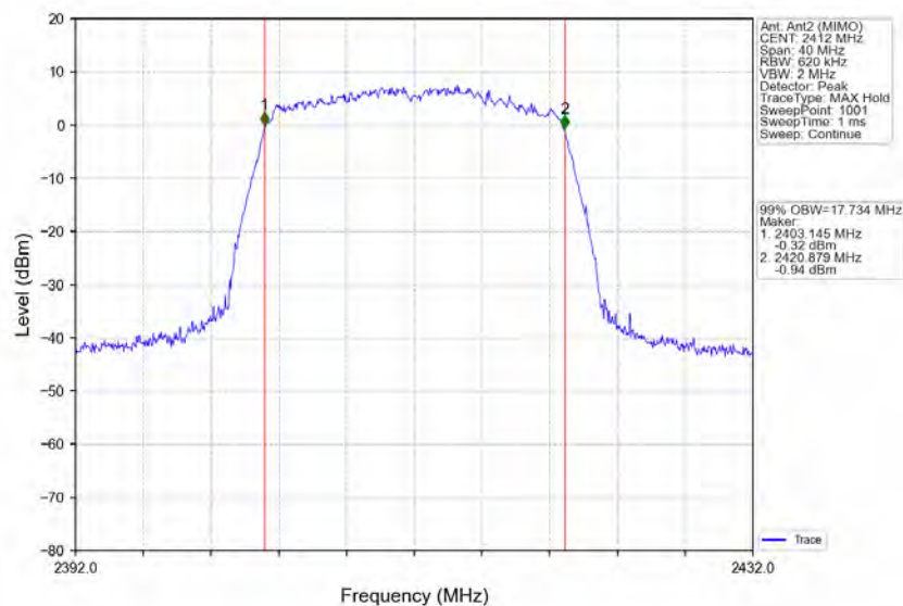
802.11n(HT20)_LCH_2412MHz_Ant2 (MIMO)_NTNV
