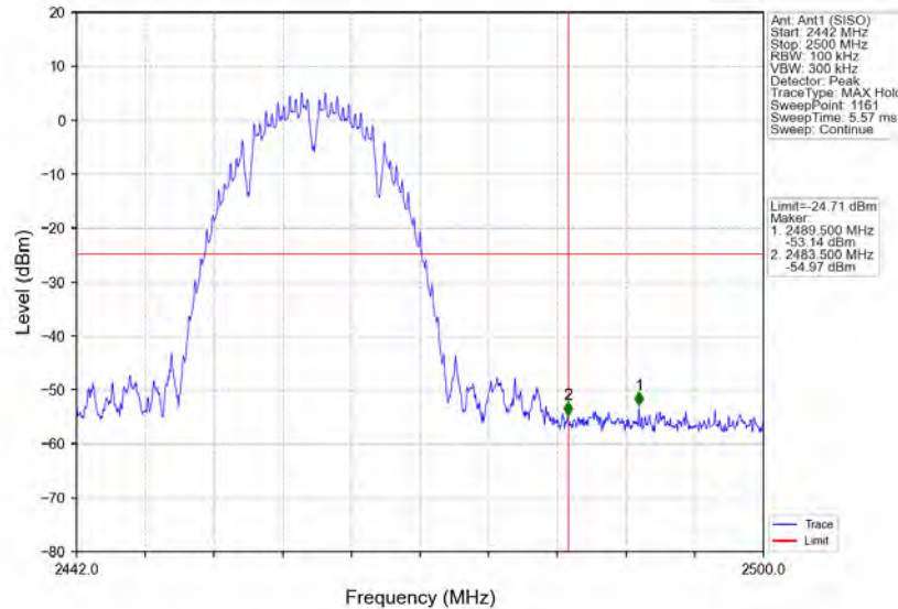
802.11b_HCH_2462MHz_Ant1 (SISO)_NTNV
