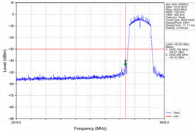
802.11n(HT20)_LCH_2412MHz_Ant1 (MIMO)_NTNV
