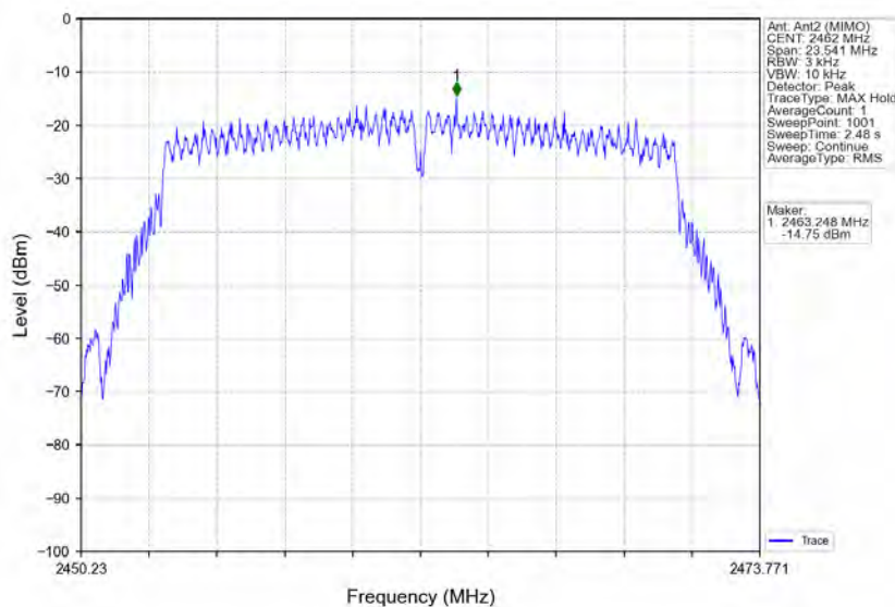
802.11n(HT20)_HCH_2462MHz_Ant2 (MIMO)_NTNV
