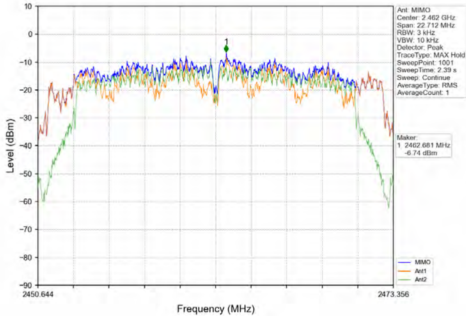
802.11n(HT20)_HCH_2462MHz_MIMO_NTNV
