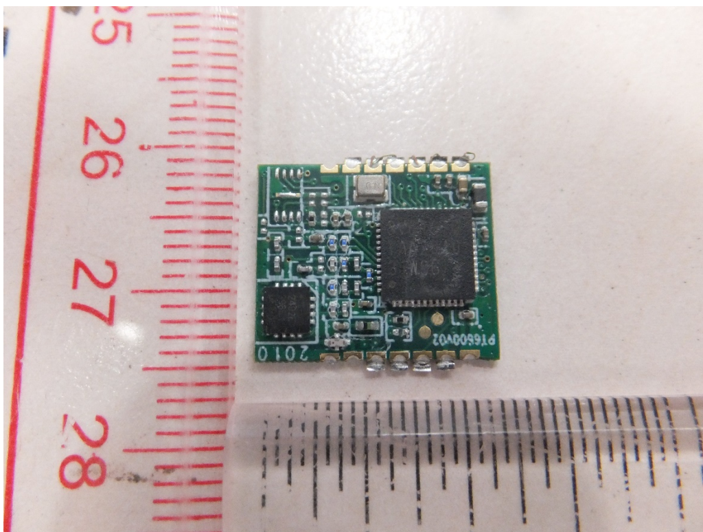
Fig. 18. WIFI module
