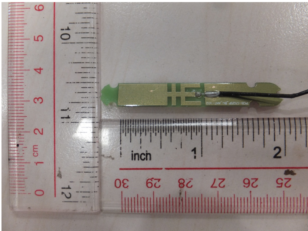
Fig. 20. WIFI antenna
