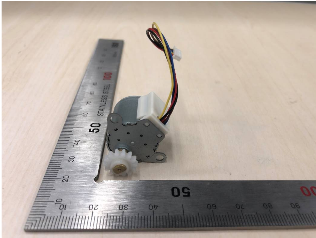
Fig. 17. Motor view
