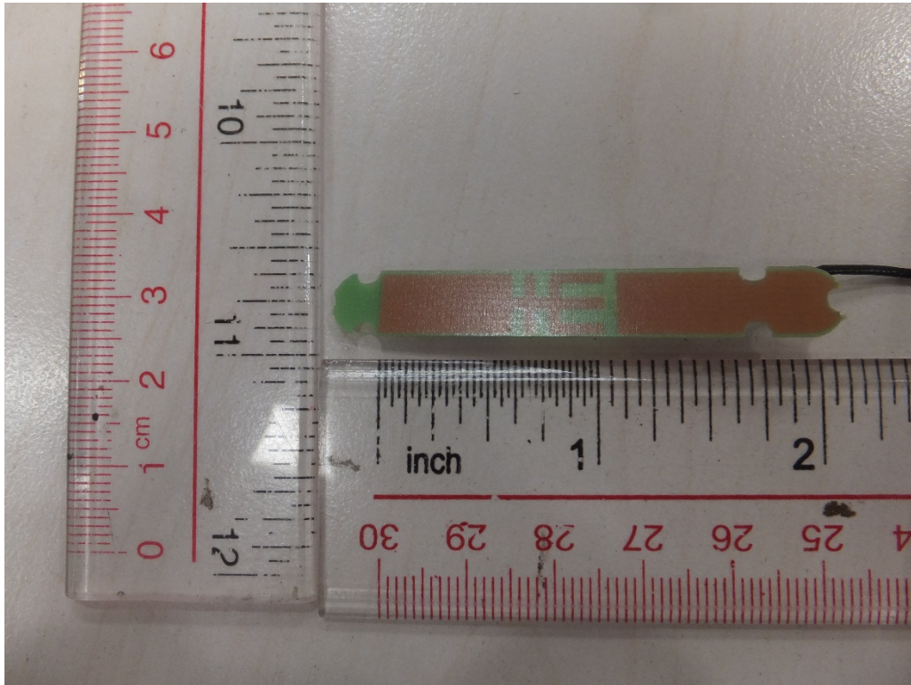
Fig. 21. WIFI antenna
