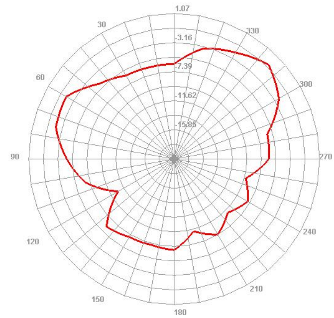
2010.000MHz E2
