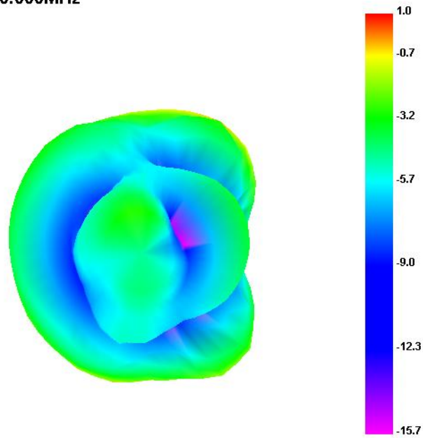
1910.000MHz
