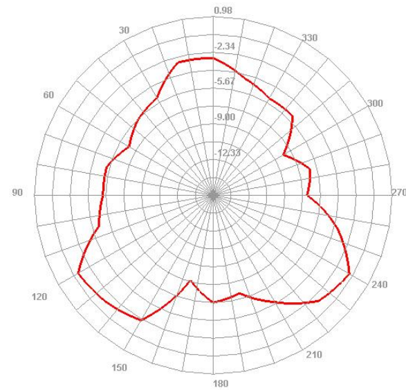
1910.000MHz E2
