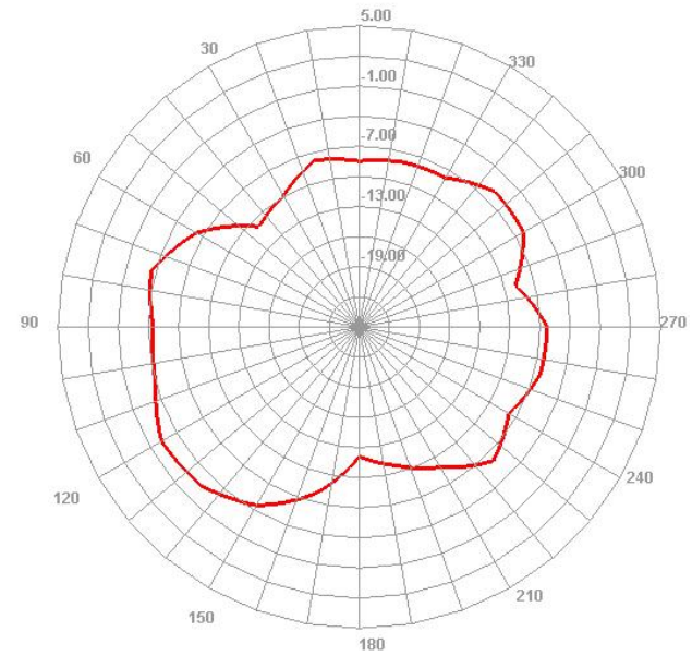
2010.000MHz H
