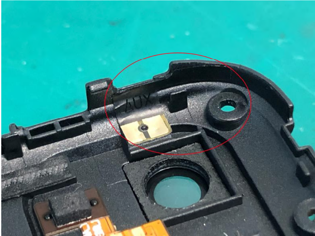
Antenna-AUX
