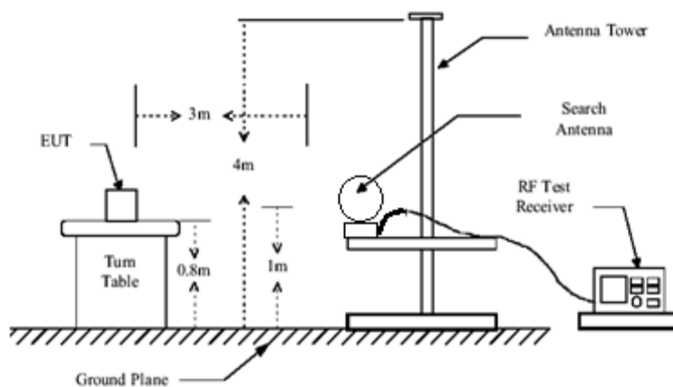
Below 1GHz(30MHz~1GHz)
