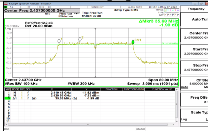
11N40SISO Ant1 2437
