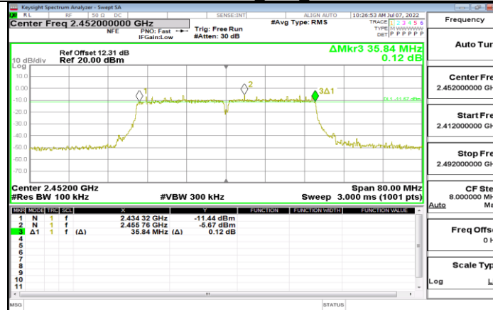
11N40SISO Ant1 2452
