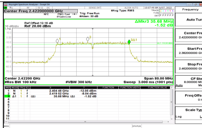
11N40SISO Ant1 2422
