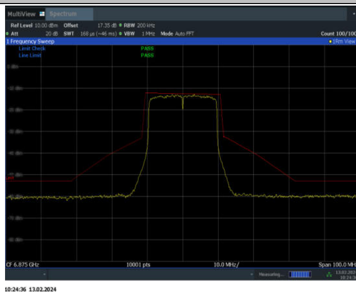
11AX20SISO_Ant7_6875
