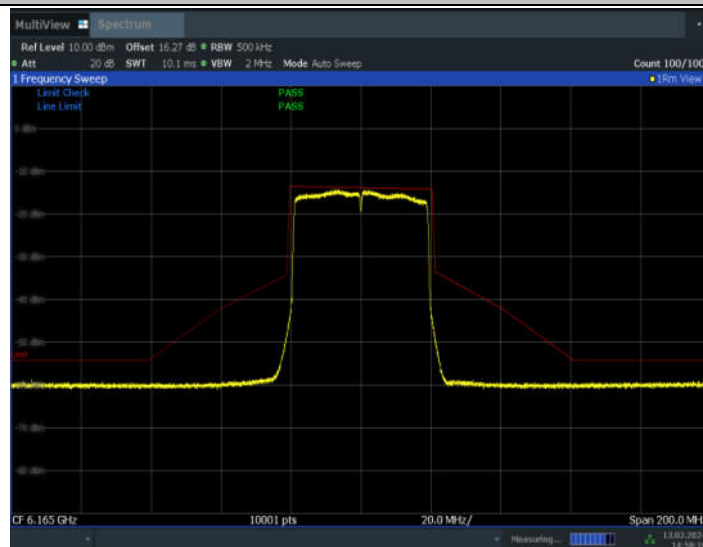
11AX40MIMO_Ant7_6165
