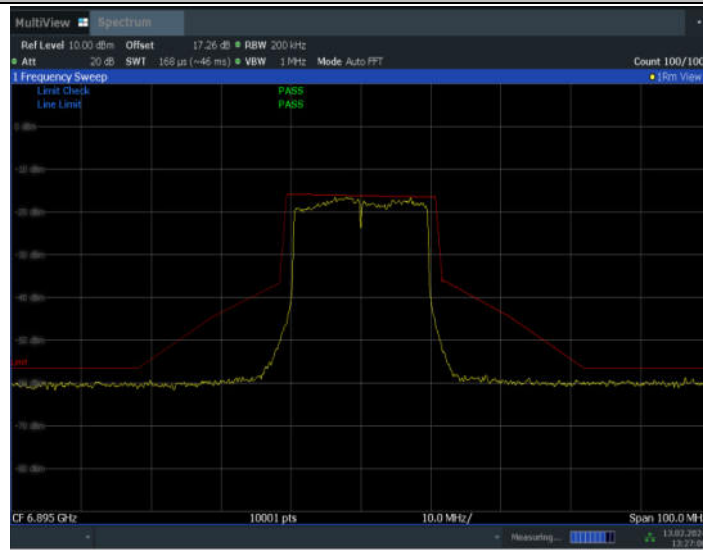
11AX20MIMO_Ant7_6895
