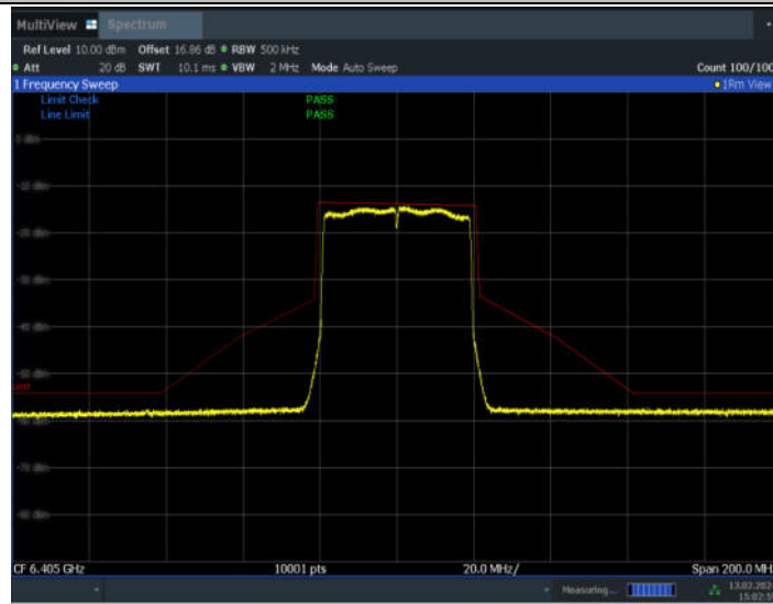
11AX40MIMO_Ant7_6405
