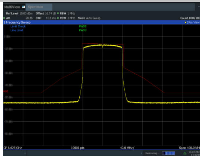
11AX80SISO_Ant7_6625
