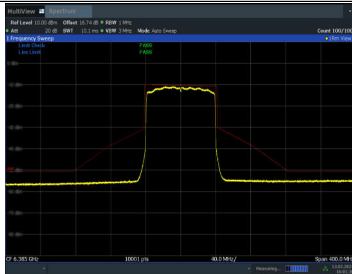
11AX80MIMO_Ant10_6385
