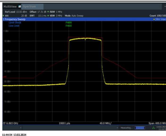
11AX80SISO_Ant7_6865
