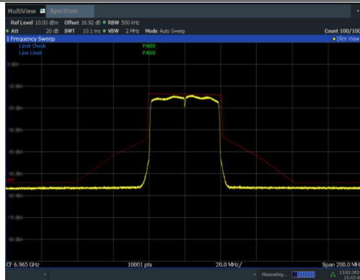
11AX40MIMO_Ant7_6965
