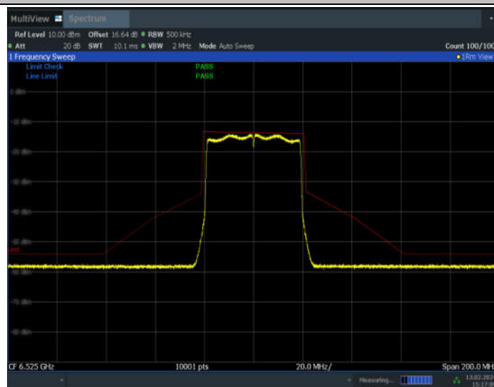
11AX40MIMO_Ant7_6525
