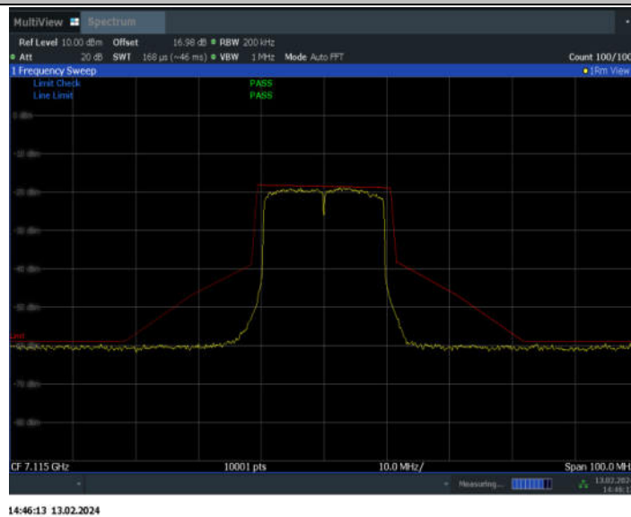
11AX20MIMO_Ant7_7115
