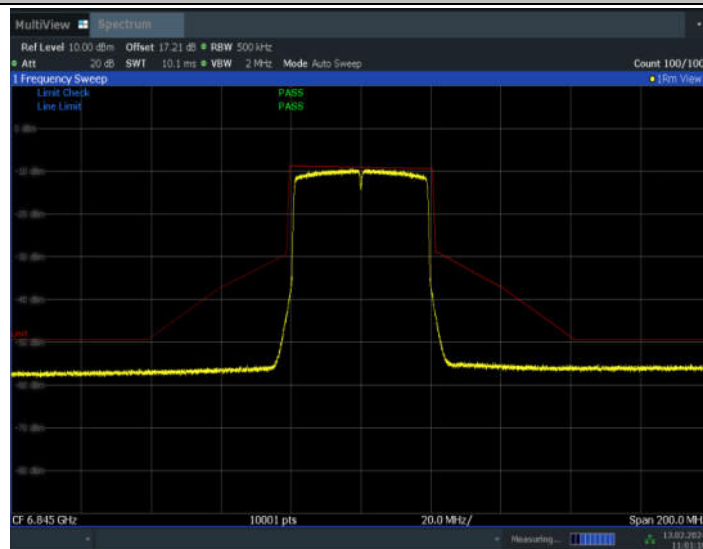
11AX40SISO_Ant7_6845
