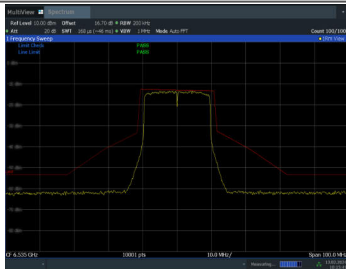
11AX20SISO_Ant7_6535
