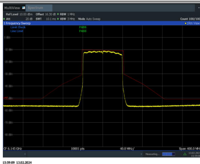
11AX80MIMO_Ant7_6145
