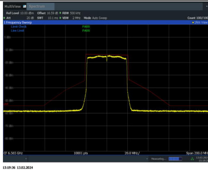
11AX40MIMO_Ant7_6565
