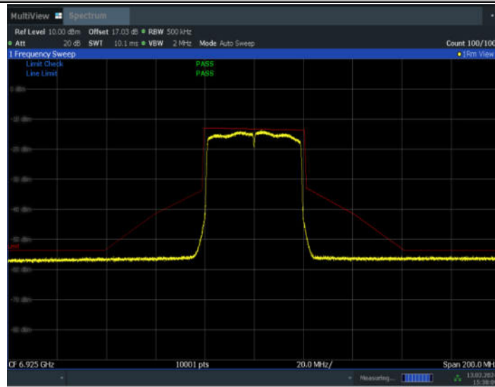
11AX40MIMO_Ant10_6925
