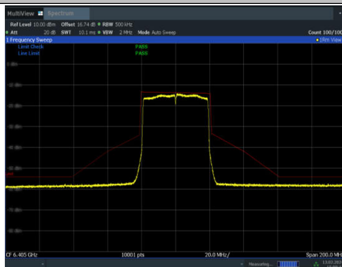
11AX40MIMO_Ant10_6405
