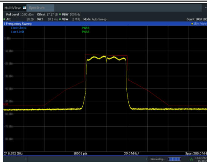
11AX40MIMO_Ant7_6925
