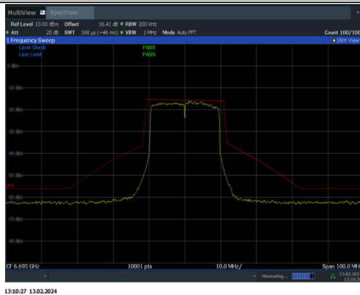
11AX20MIMO_Ant7_6695
