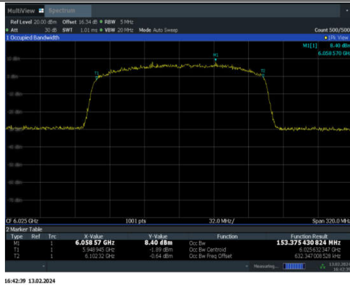
11AX160MIMO_Ant7_6025
