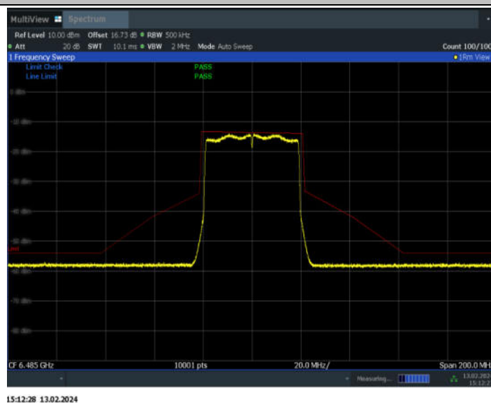
11AX40MIMO_Ant7_6485
