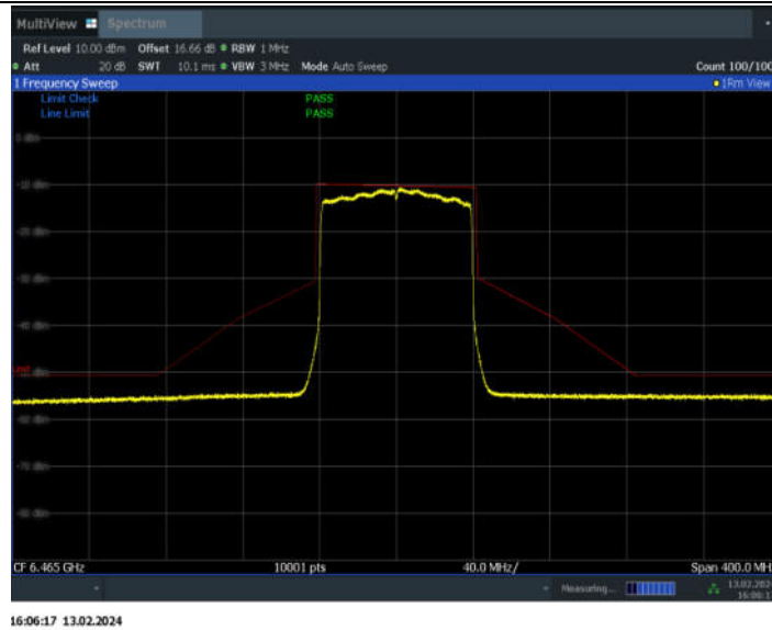
11AX80MIMO_Ant7_6465
