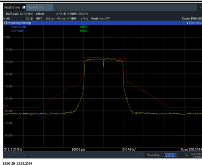
11AX20MIMO_Ant10_6515
