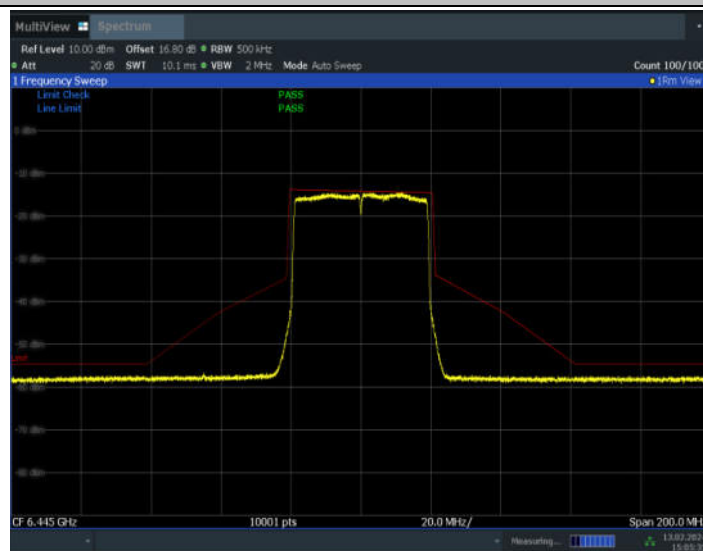
11AX40MIMO_Ant10_6445
