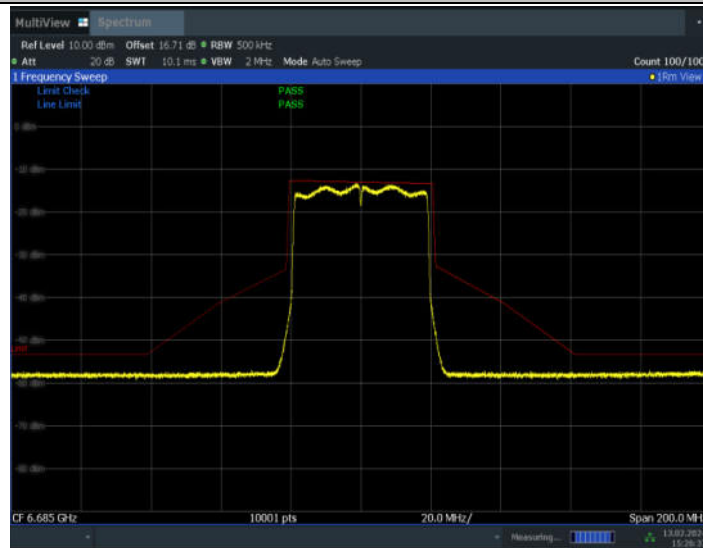
11AX40MIMO_Ant7_6685
