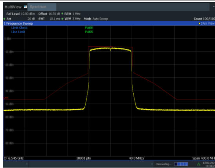
11AX80SISO_Ant7_6545
