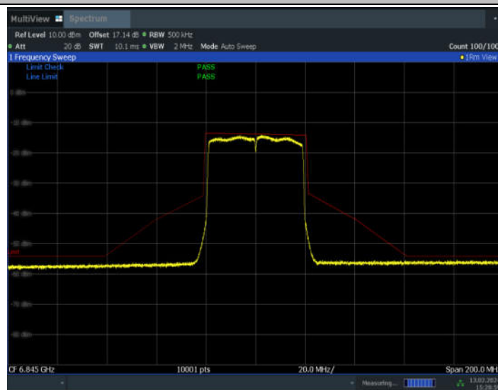
11AX40MIMO_Ant10_6845
