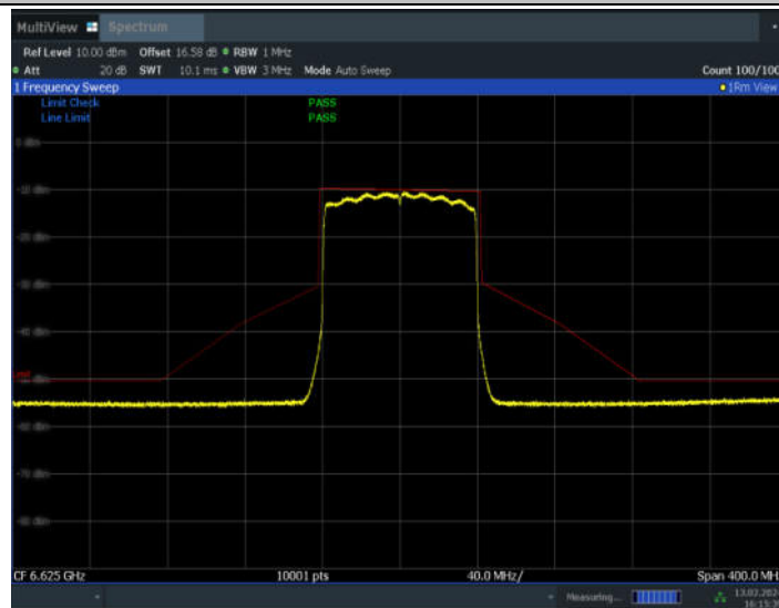
11AX80MIMO_Ant10_6625
