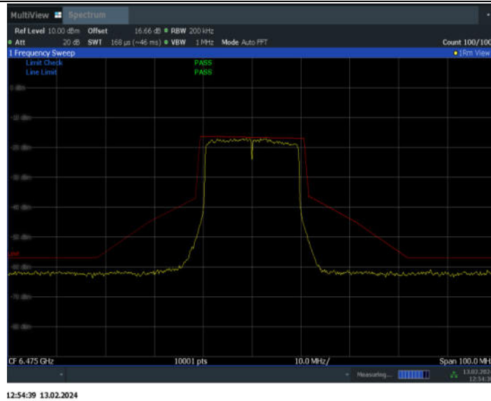
11AX20MIMO_Ant7_6475
