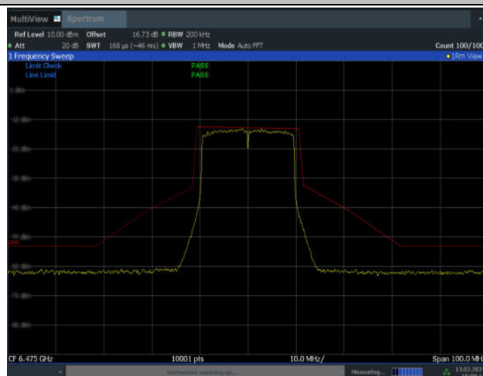
11AX20SISO_Ant7_6475
