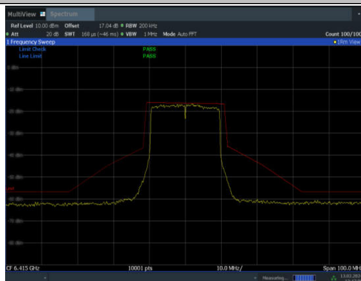
11AX20MIMO_Ant7_6415
