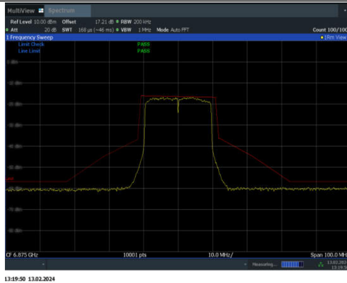
11AX20MIMO_Ant7_6875
