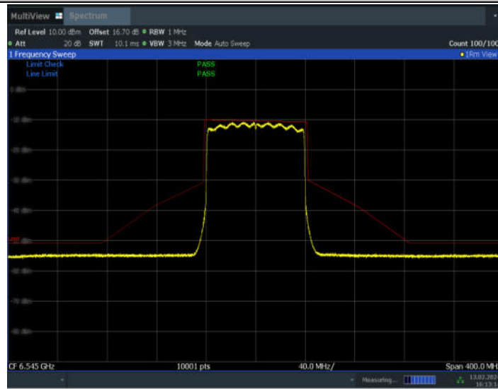
11AX80MIMO_Ant7_6545
