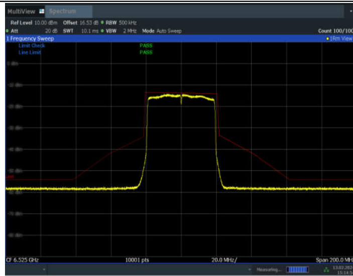
11AX40MIMO_Ant10_6525
