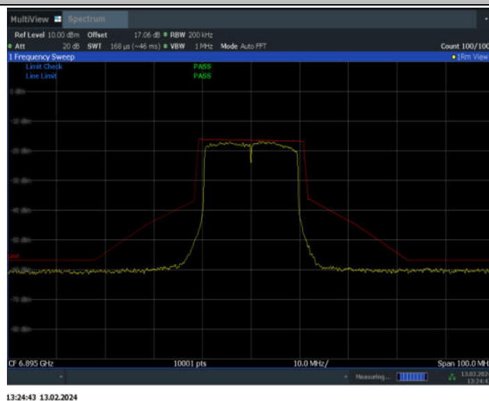
11AX20MIMO_Ant10_6895
