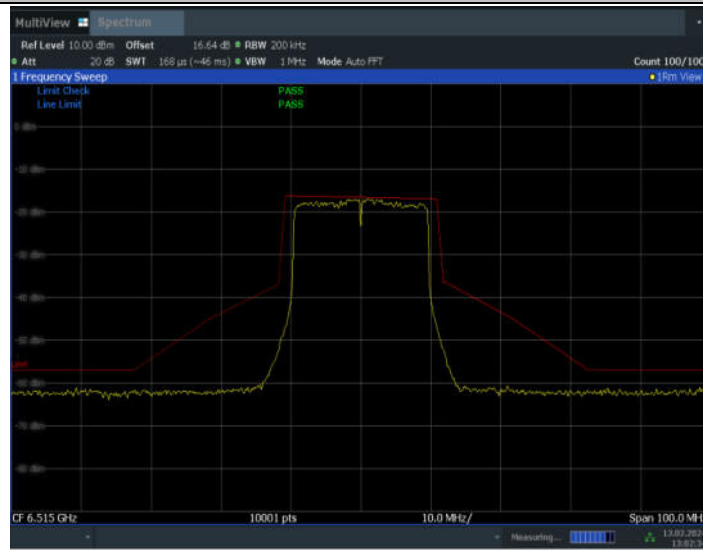
11AX20MIMO_Ant7_6515
