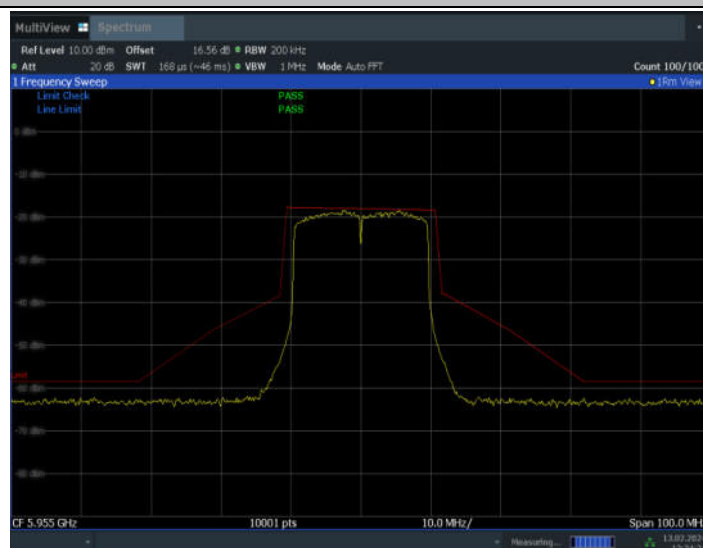
11AX20MIMO_Ant10_5955
