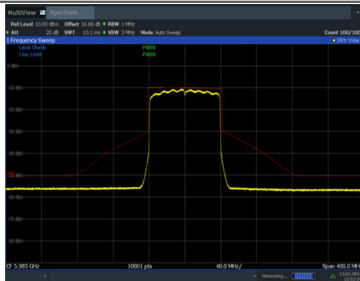
11AX80MIMO_Ant10_5985
