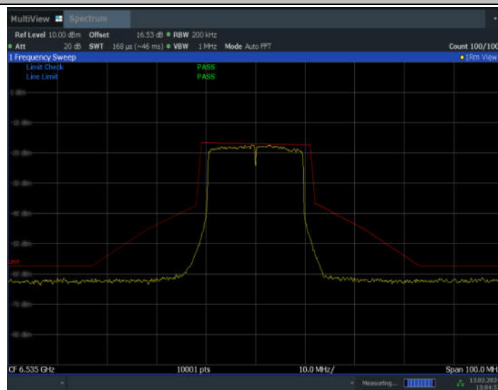
11AX20MIMO_Ant10_6535
