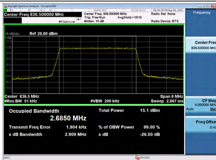
Band5-3MHz-QPSK-20635-15RB#0
