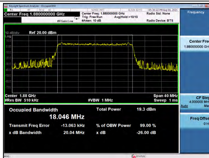
Band2-20MHz-16QAM-19100-100RB#0
