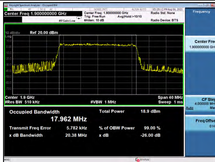
Band2-20MHz-16QAM-18700-100RB#0
