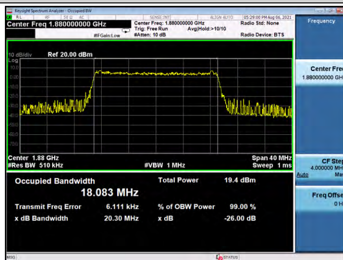
Band2-20MHz-QPSK-19100-100RB#0
