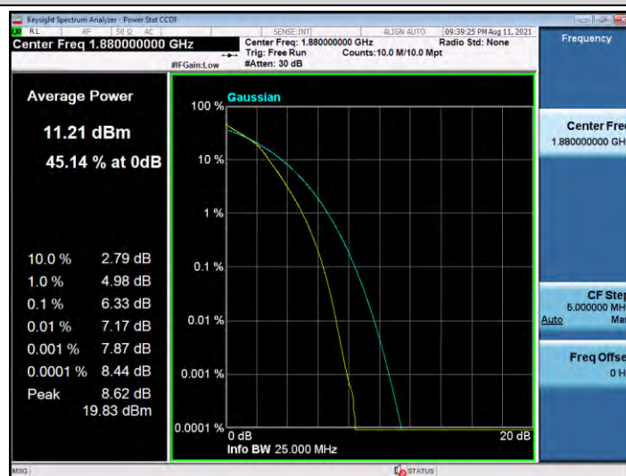
Band2-20MHz-16QAM-19100-100RB#0
